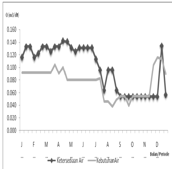
Gambar 2. Neraca Air Bendung Sumber Buntu
