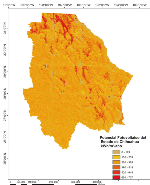
Figura 3. Potencial fotovoltaico del estado de Chihuahua.
