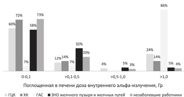
Рис. 4. Распределение работников изучаемой когорты в зависимости от поглощенных в печени доз внутреннего альфа-излучения
