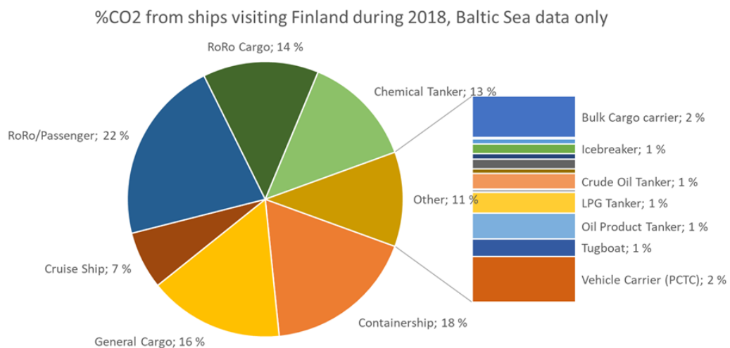
Liite 2. Vuoden 2018 aikana Suomen satamissa käyneiden alusten CO2-päästöt Itämerellä alusluokittain. Kuusi suurinta alusluokkaa tuottaa yli 90 % kokonaispäästöistä.
