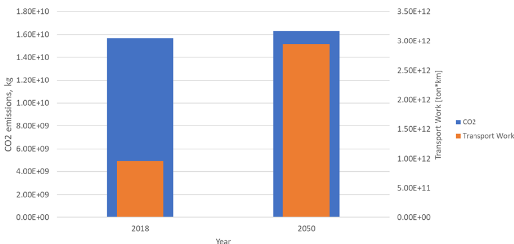
Kuvio 11 Itämeren meriliikenteen CO 2 -päästöt ja kuljetussuorite vuosina 2018 ja ennuste vuodelle 2050 huomioiden EEDI-säännöt, alusten koon kasvu ja alusmäärissä tapahtuvat muutokset. Vuoden 2018 CO 2 -päästö oli 15,7 miljoonaa tonnia ja ennuste vuoden 2050 laivaliikenteen CO 2 -päästöiksi on 16,3 miljoonaa tonnia.
