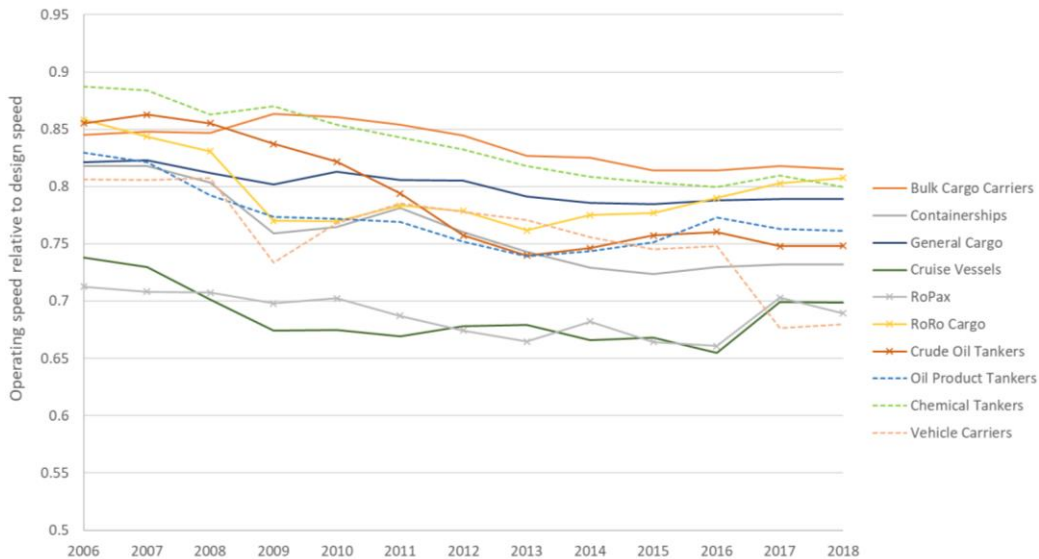
Kuvio 14 Itämerellä purjehtivien alusten keskimääräiset operointinopeudet v. 2006–2018 (HELCOM Maritime 19, 2019) verrattuna alusten suunnittelunopeuteen
