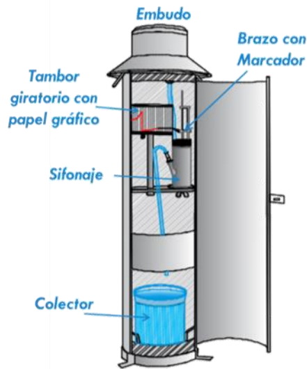
Figura 4 El fluviógrafo
