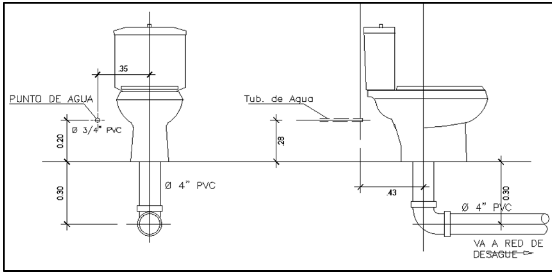
Figura 24: Tuberías
