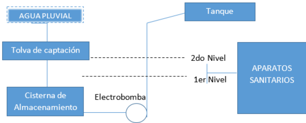
Figura 14 Esquema de captación y conducción de Agua pluvial.
