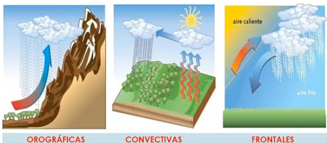
Figura 6 Tipos de precipitación
