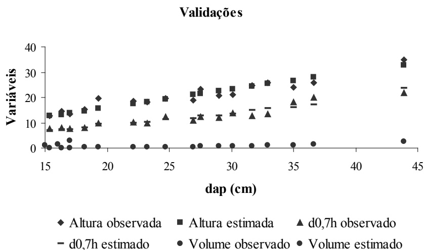
FIGURA 3: Valores observados e estimados da altura total, d 0,7h e volume usado para validação das equações.
