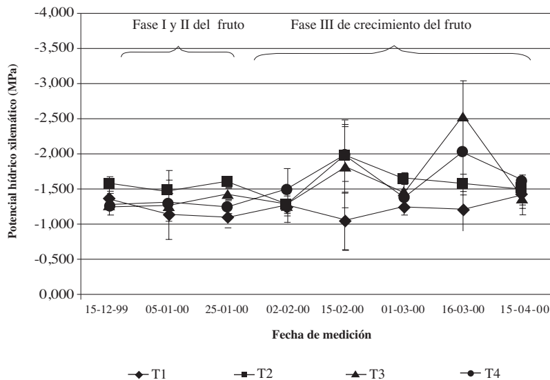
Figura 2. Efecto de los tratamientos de riego sobre el potencial hídrico xilemático medido a mediodía (MPa) en la temporada 1999-2000.
