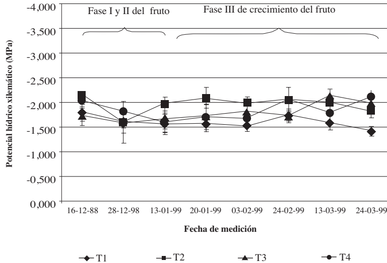
Figura 1. Efecto de los tratamientos de riego sobre el potencial hídrico xilemático medido a mediodía (MPa) en la temporada 1998-1999.
