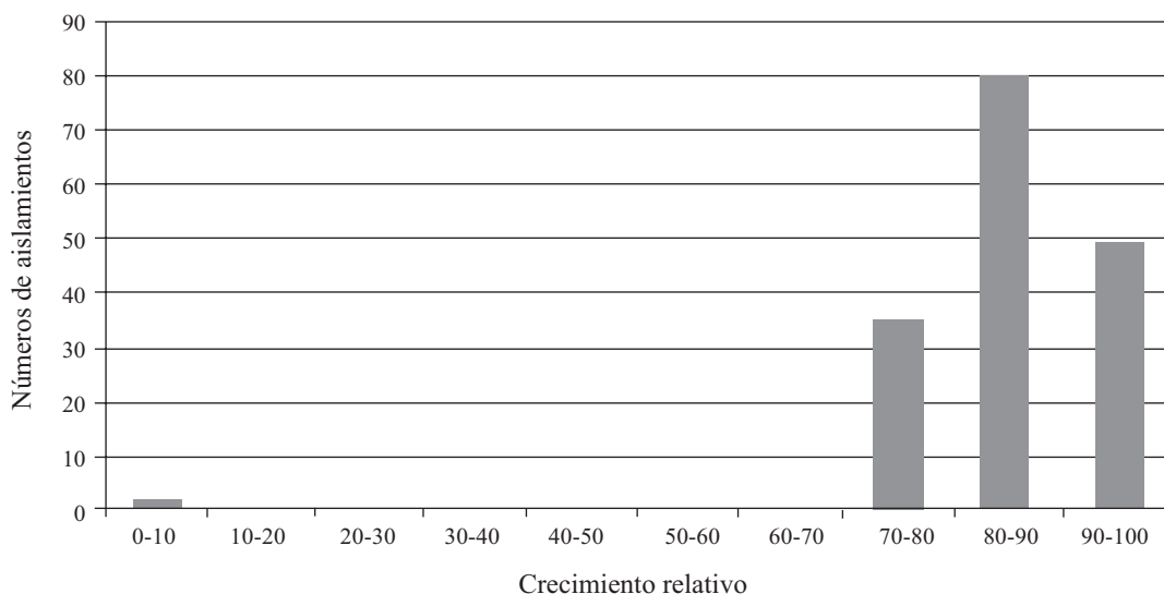
Figura 1. Distribución de frecuencias en función del porcentaje de crecimiento relativo (respecto colonia testigo) de 164 aislamientos de Phytophthora infestans sobre agar centeno B y 10 mg L -1 de metalaxil de Regiones IV y V. Temporada 1999.
