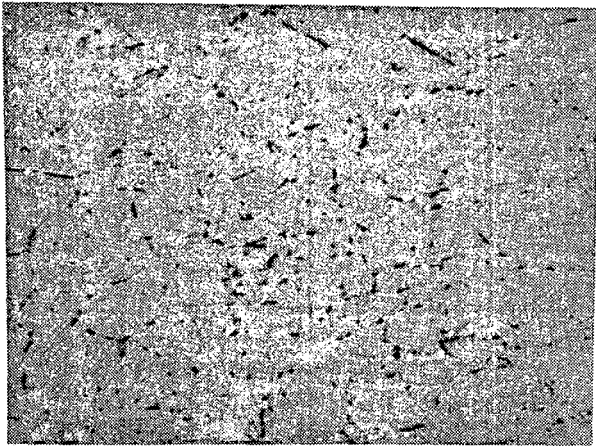
Figura 1: 304 Martensítico. X 100
