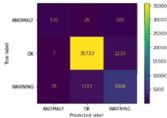
Fig. 4. Matriz de confusión arrojada como resultado de evaluar el perceptrón multi-capa con el dataset de prueba empleando cross-validation .
