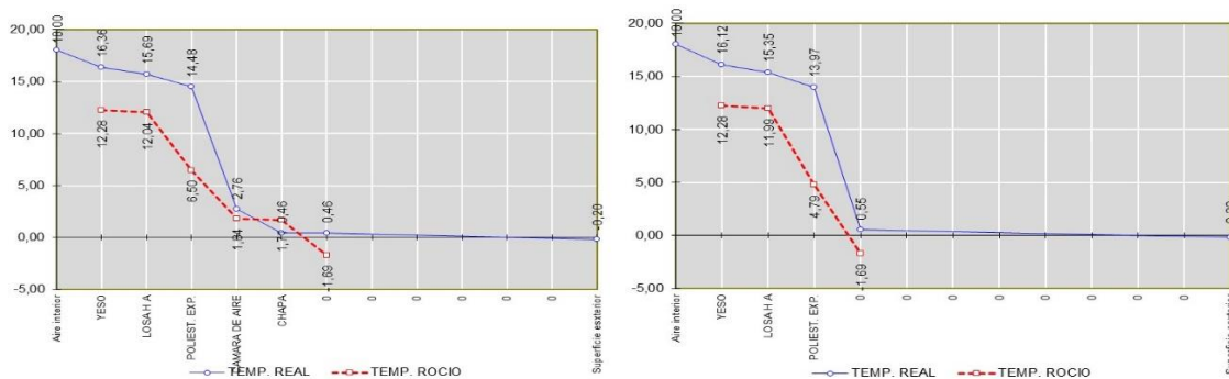
Figura 6: Verificación de riesgo de condensación para el techo de losa con cubierta de chapa con cámara de aire: fig. izquierda: cerrada y fig. derecha: abierta.
