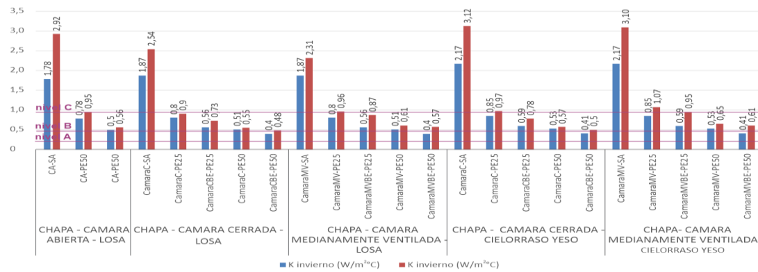
Figura 5: Variación de los valores de K de las soluciones constructivas de techos de chapa, sobre losa y sobre cielorraso de yeso, según grado de ventilación de la cámara de aire.
