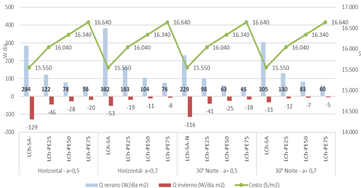
Figura 15: Variación de la carga térmica y costos del techo de chapa sobre losa con cámara cerrada.
