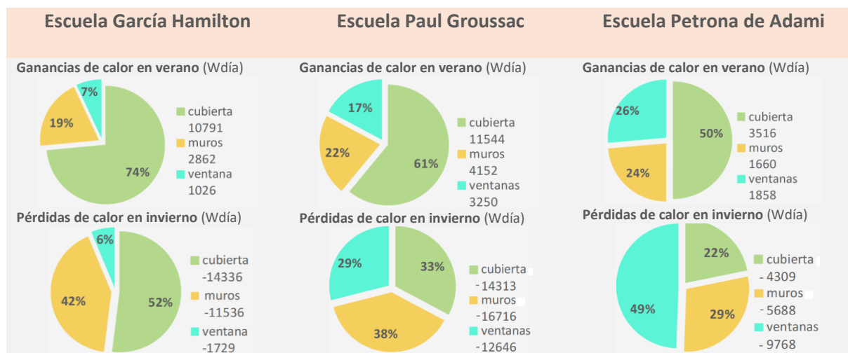
Figura 2: Carga térmica total a través de cada uno de los elementos de la envolvente de aulas prototípicas de escuelas de S.M. de Tucumán
