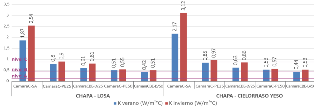
Figura 4: Variación de los valores de K de las soluciones constructivas de techos de chapa, sobre losa y sobre cielorraso de yeso, según grado de aislamiento térmico
