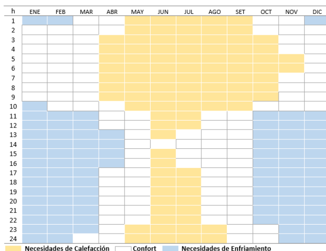
Figura 1: Diagrama de solicitudes térmicas para el confort para S.M. de Tucumán
