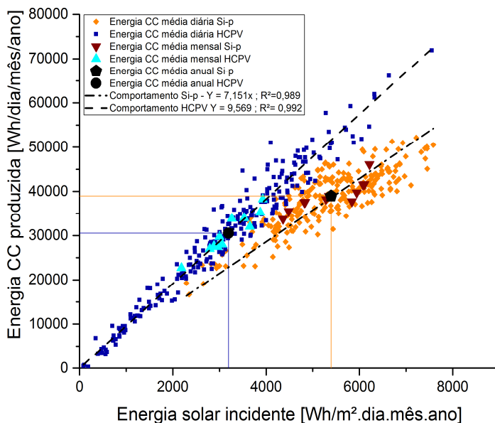
Figura 6. Comparação entre o comportamento da produção de energia CA dos sistemas HCPV e policristalino.
