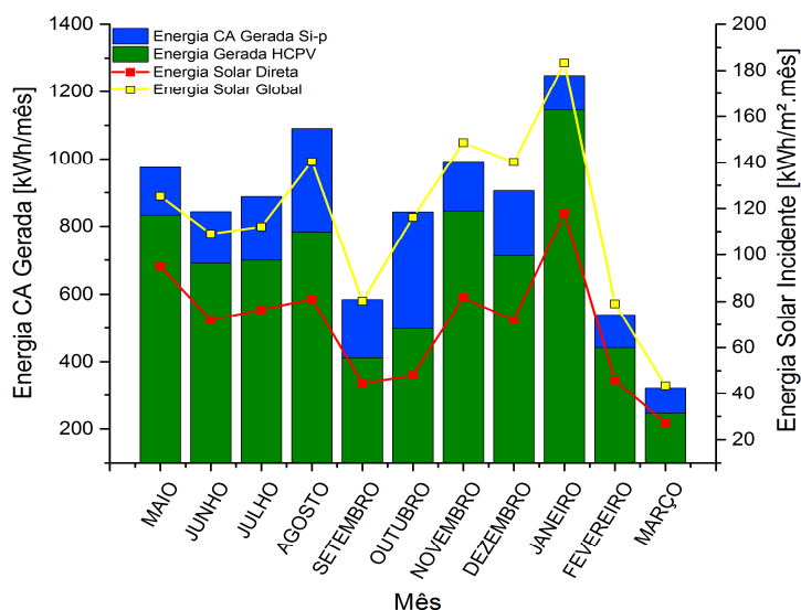
Figura 7. Comparação entre a energia CA gerada por cada sistema.
