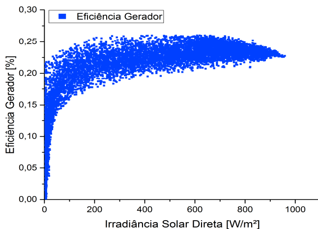
Figura 5. Eficiência do gerador fotovoltaico do sistema HCPV FAE-UFPE.
