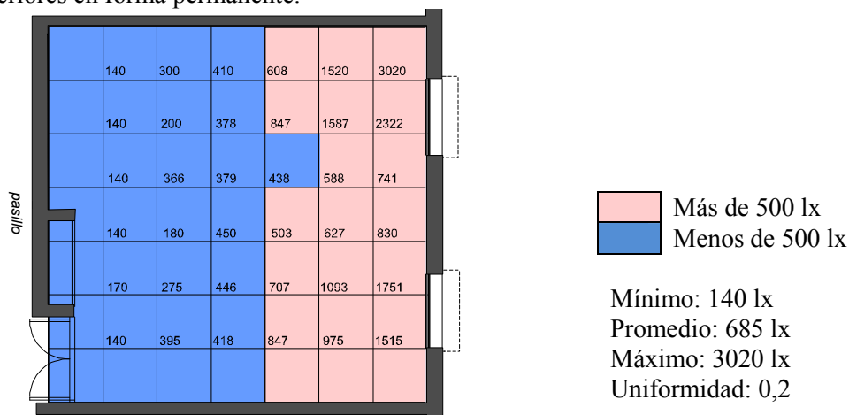
Figura 10: Valores de iluminancia registrados in situ, bajo condiciones de cielo claro
