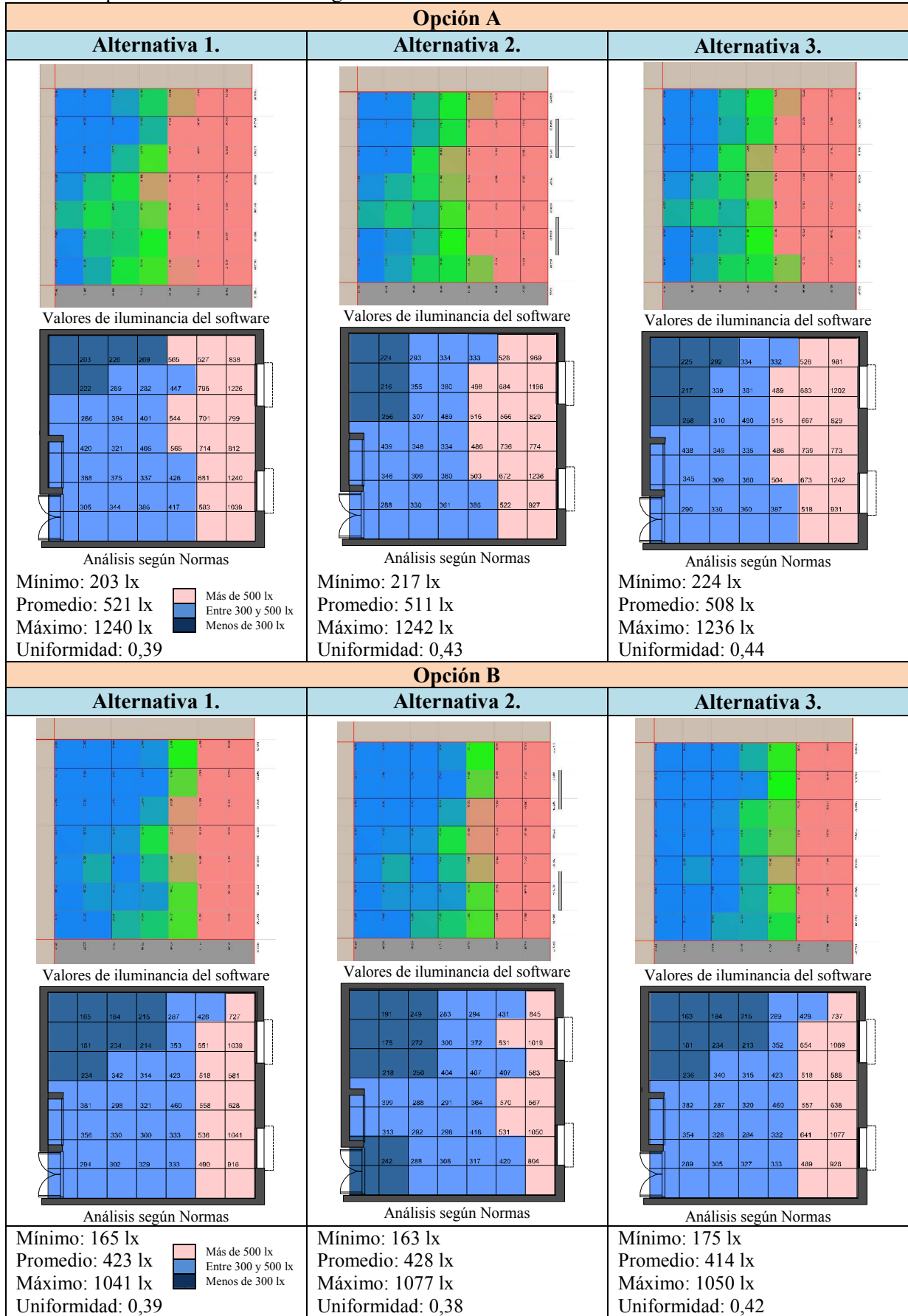
Figura 16: Resultados de la simulación lumínica del aula para las diferentes soluciones de diseño.
