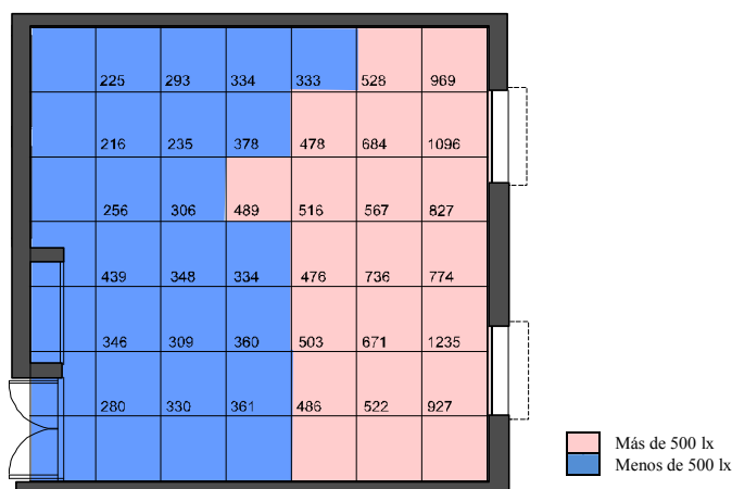
Figura 17: Valores de iluminancia para Junio 11:00 hs
