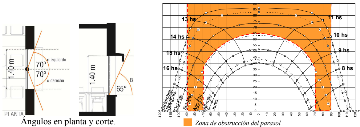
Diagrama de trayectoria solar en superposición a diagrama de visión de bóveda para la orientación norte.
