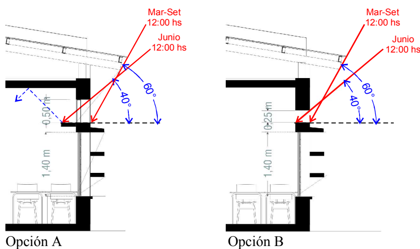
Figura 12: Ángulos de obstrucción solar de las ventanas superiores
