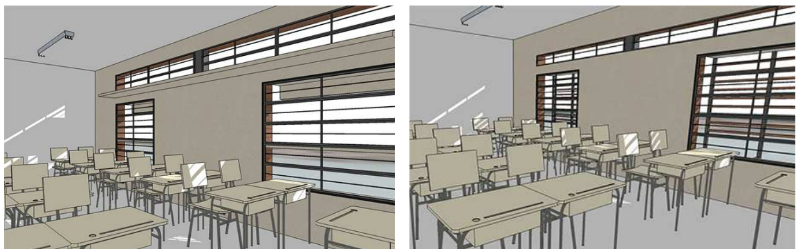
Figura 14: Vistas interiores de las opciones A y B de ventanas superiores.
