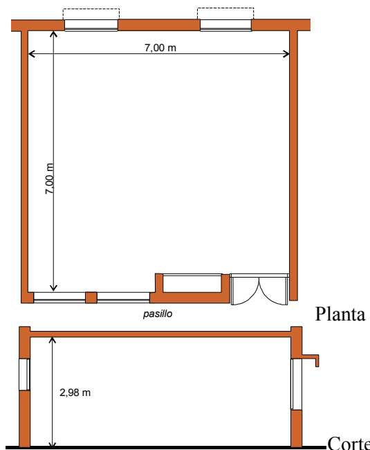
Figura 7: Características del aula seleccionada para el análisis
