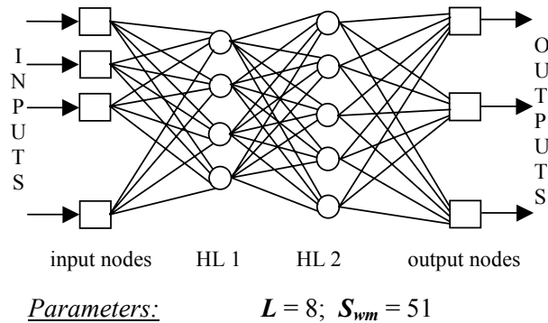
Fig. 2. Parameters definition of an ANN
