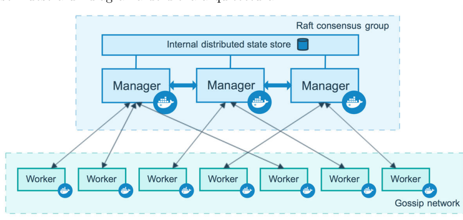
Figura 3: Arquitectura de Docker Swarm
