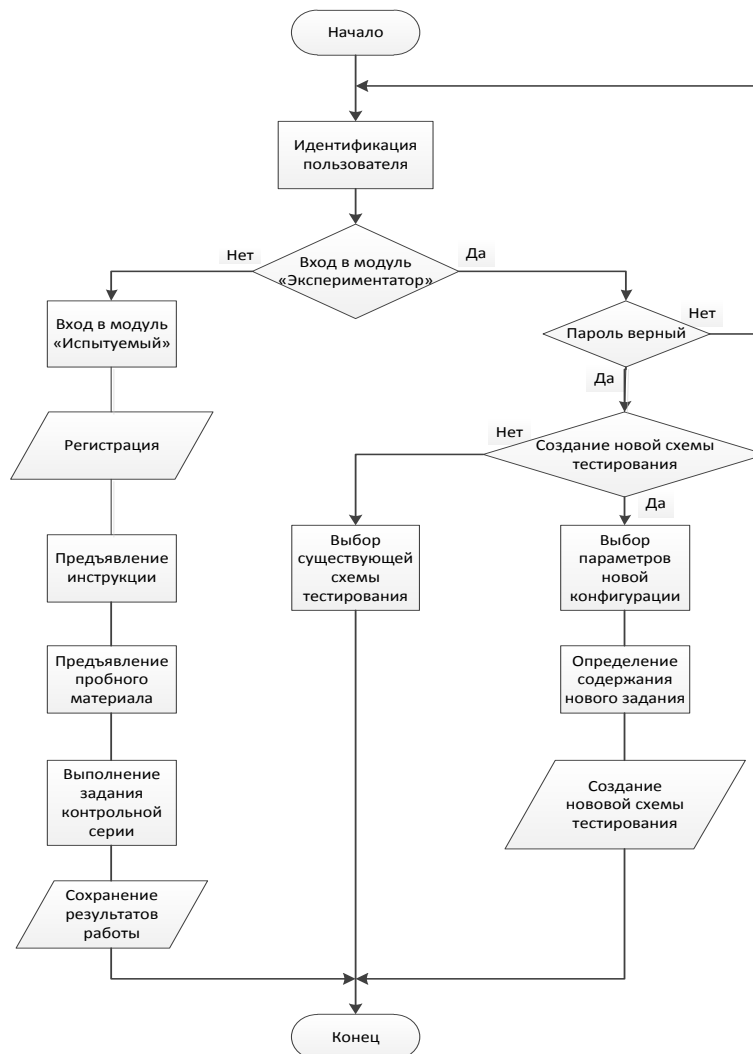
Рис. 2. Блок-схема алгоритма работы программы
