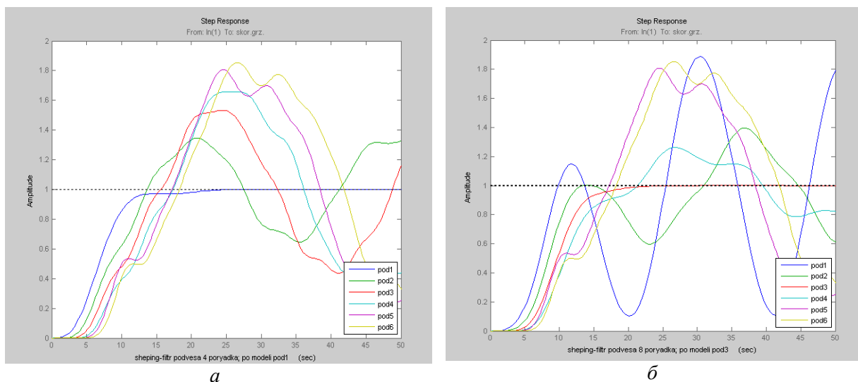
Рис. 5. Переходные характеристики по скорости конечного звена для шести случаев с применением шейпинг-фильтра с разным порядком: а – шейпинг-фильтр четвертого порядка; б – шейпинг-фильтр восьмого порядка
