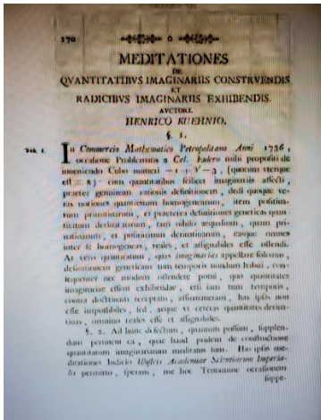
Figs. 9, 10. Meditationes de quantitativus imaginariis construendis et radicibus imaginariis exhibendis. Novi Commentarii Academiae Scientiarum Imperialis Petropolitanae 3 (1753), front page and the complex numbers diagram.
