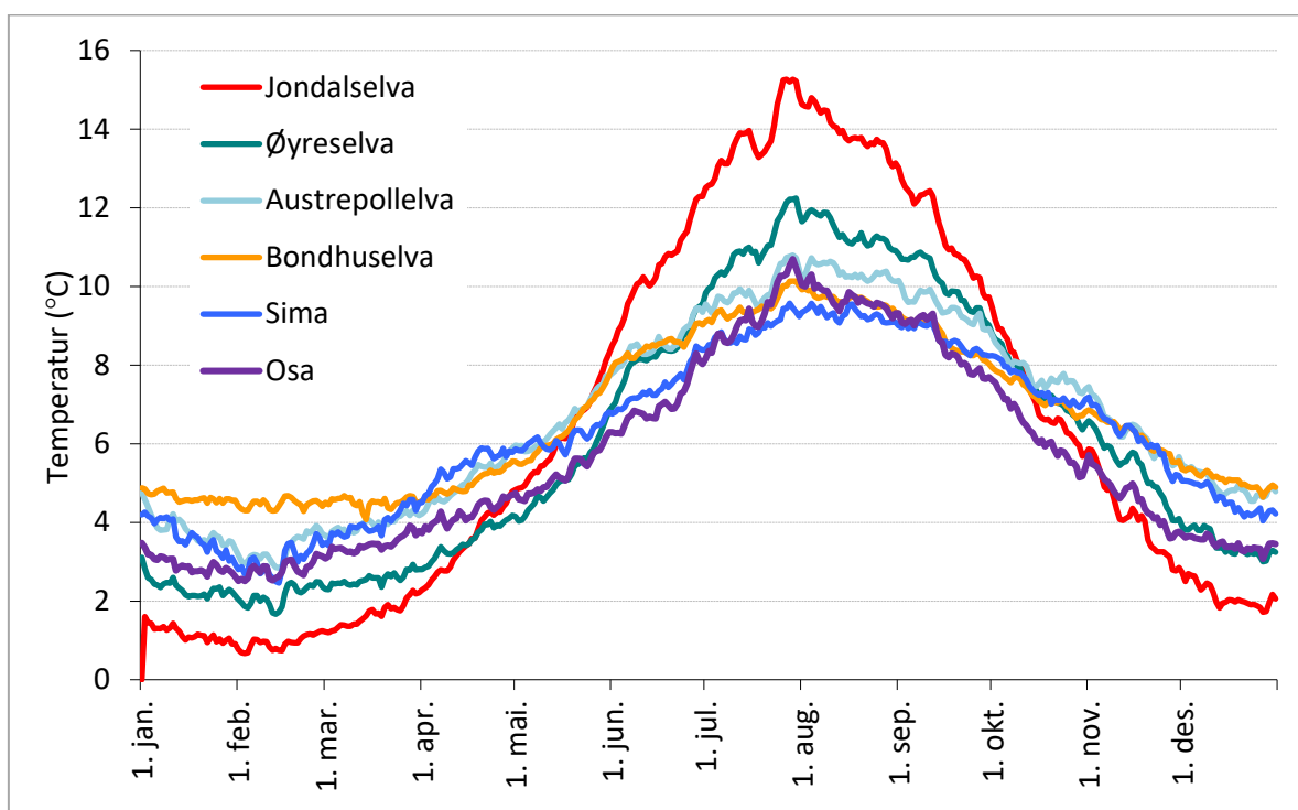
Figur 4. Gjennomsnittlig vanntemperatur på døggnivå fra de seks regulerte elvene i Hardanger i perioden 2007-2021.
