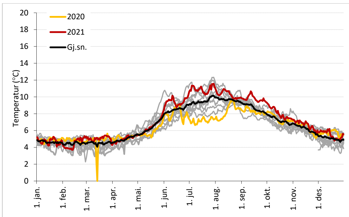
Figur 29. Døgnmiddeltemperatur i Bondhuselva i perioden 2008-2021. Data fra 2020 og 2021 er markert i farger, mens de grå linjene indikere data fra enkeltår tidligere i perioden.
