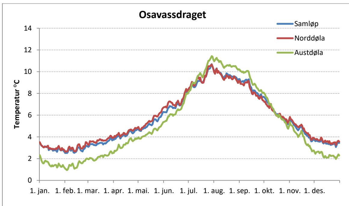
Figur 10. Døgnmiddeltemperaturer (gjennomsnitt for døgn) i de ulike vassdragsavsnittene i Osavassdraget i perioden 2008-2021.
