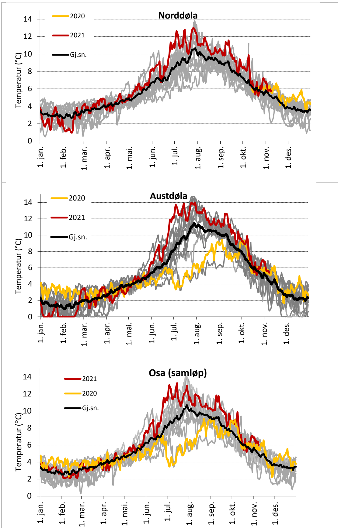
Figur 11. Døgnmiddeltemperatur i Norddøla (øverst), Austdøla (midten) og samløpet (nederst) i 2008-2021. Data for 2020 og 2021 er markert i farger, mens grå linjer er data for de enkelte år tidligere i perioden. Data fra deler av 2020 mangler i Norddøla.
