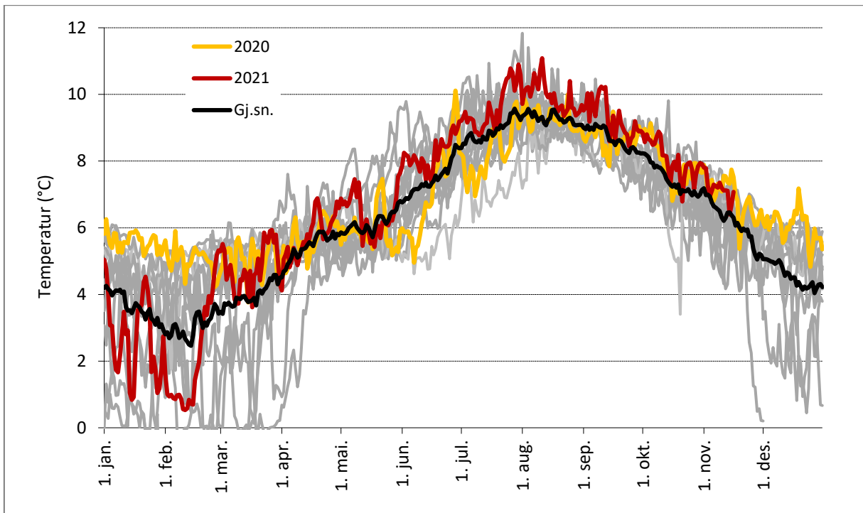
Figur 6. Døgnmiddeltemperaturer fra loggere i Sima i perioden 2008-2021. Data for 2020 og 2021 er markert i farger, mens grå linjer er data for de enkelte år tidligere i perioden. Temperaturer under 0 grader tyder på at loggeren ved flere anledninger har vært tørrlagt i perioder på vinteren.
