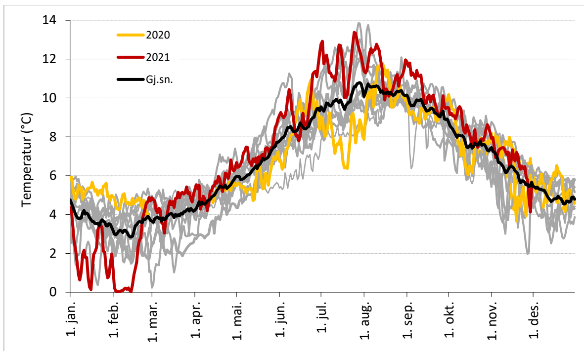
Figur 25. Døgnmiddeltemperatur i Austrepolluelva i perioden 2008-2021. Data fra 2020 og 2021 er markert i farger, mens de grå linjene indikere data fra enkeltår tidligere i perioden.
