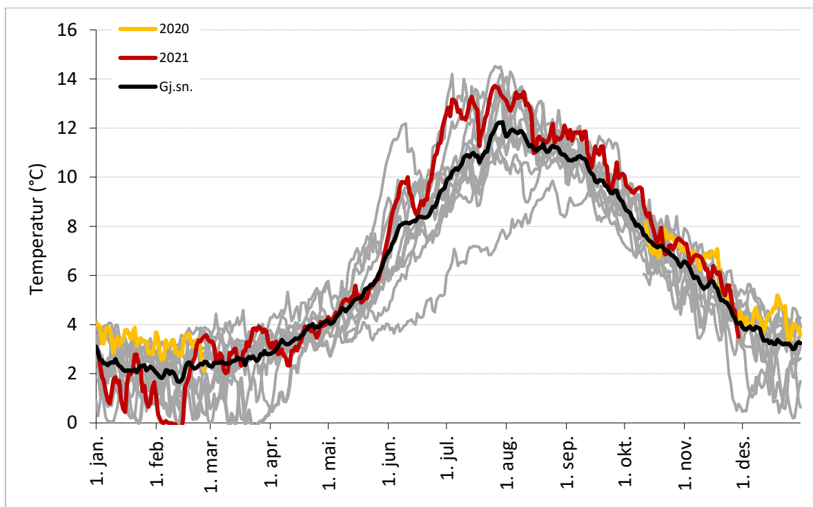
Figur 21. Døgnmiddel vanntemperatur i Øyreselva i perioden 2008-2021. Data for 2020 og 2021 er markert i farger, mens grå linjer er data for de enkelte år tidligere i perioden.
