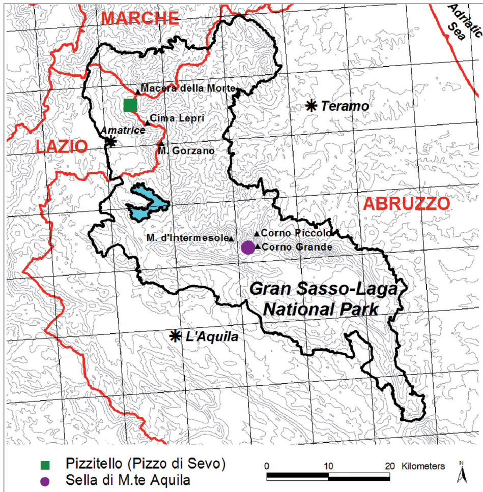
Fig. 1 - Il territorio del Parco Nazionale Gran Sasso-Monti della Laga con l'ubicazione delle popolazioni di Vaccinium gaultherioides
