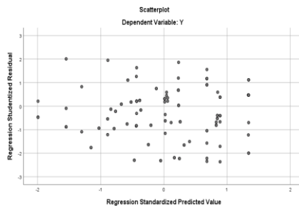
Gambar 2. Uji Heteroskedastisitas
