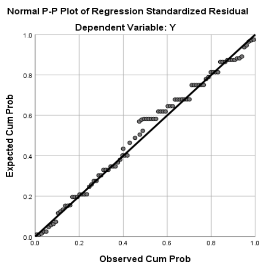
Gambar 1. Uji Normalitas
