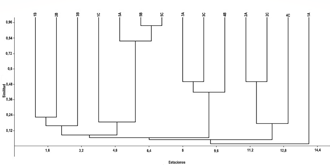
Figura 3. Análisis de similitud de Jaccard para las estaciones de muestreo basado en las abundancias.
