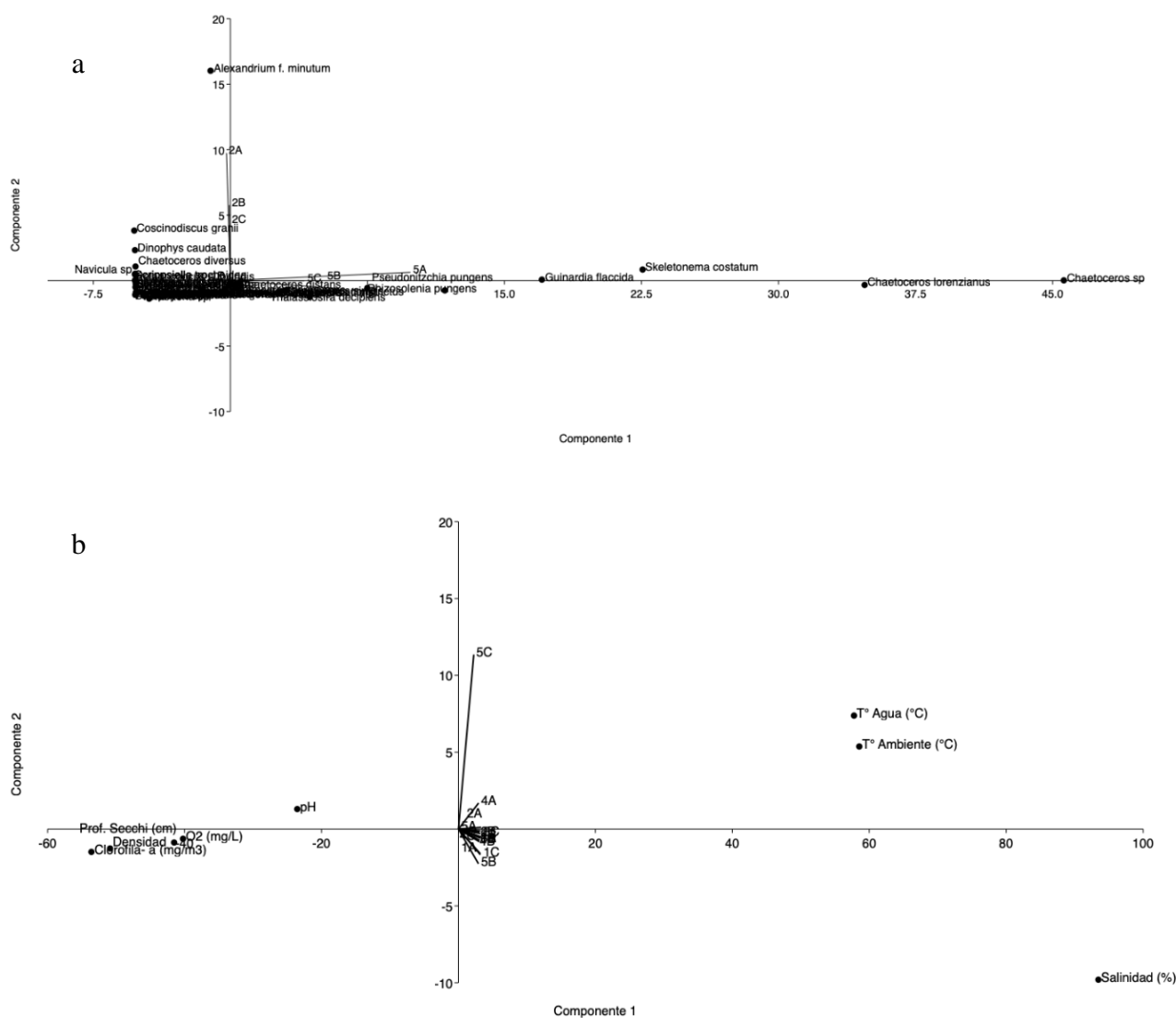
Figura 4. Análisis de componentes principales para estaciones y especies (a), y para estaciones y fisicoquímicos (b).
