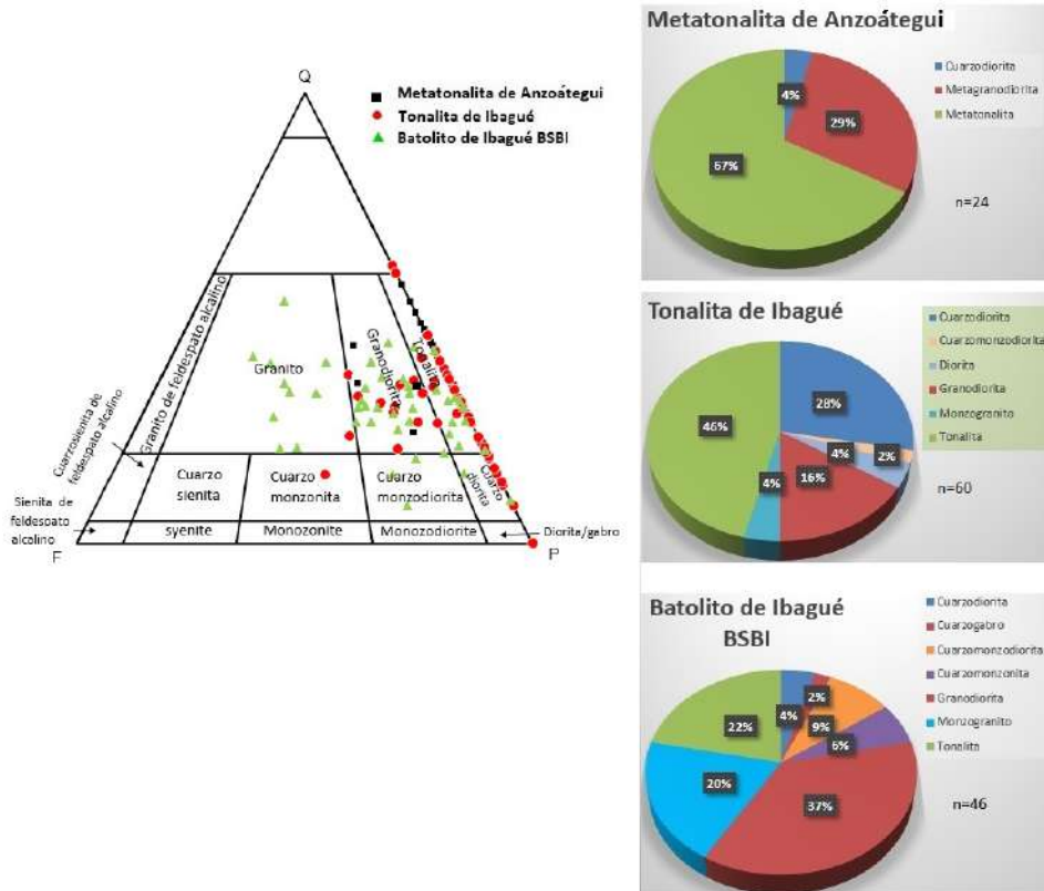
Figura 6. Clasificación petrográfica de las muestras de la Metatonalita de Anzoátegui, la Tonalita de Ibagué y el batolito de Ibagué, y composición litológica en porcentaje por bloques y por unidad.
