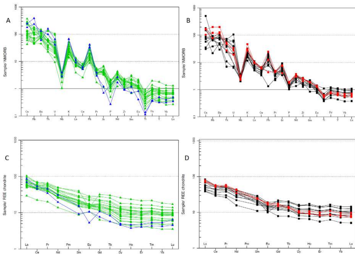
Figura 14. Principales características geoquímicas de las rocas de la Metatonalita de Anzoátegui y la Tonalita de Ibagué (rojo y negro, respectivamente) y batolito de Ibagué (verde y azul, de las cuales las azules presentan alteración potásica). A. y B. Diagramas de elementos trazas normalizados al NMORB según los valores de Sun y McDonough (1989). C. y D. Patrones de elementos de tierras raras respecto al condrito según los valores de Nakamura (1974).
