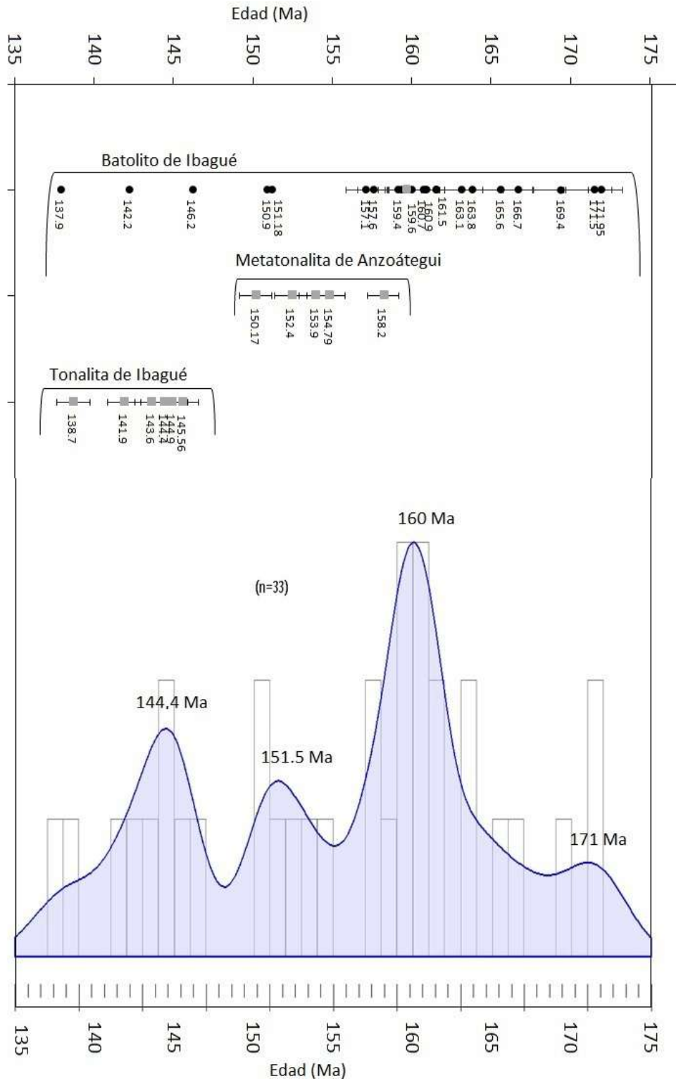
Figura 11. Distribución de edades en el batolito de Ibagué, la Metatonalita de Anzoátegui y la Tonalita de Ibagué y diagrama de estimación de densidad de Kernel a partir de las edades de cristalización U-Pb.
