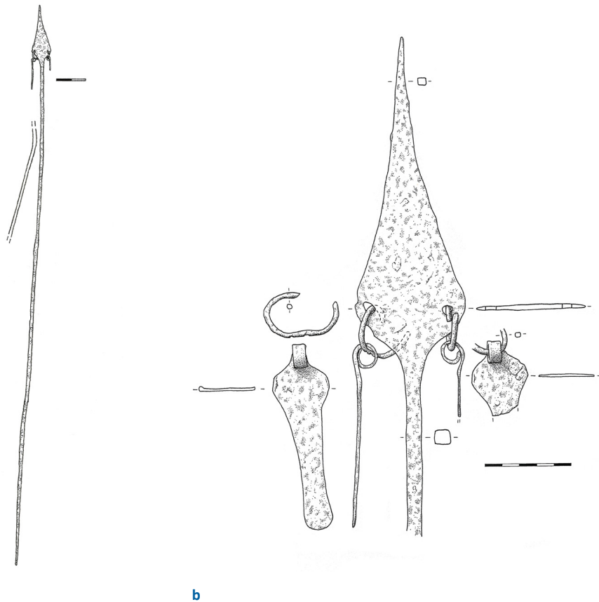
9 Boğazköy, Hattuša. Standarte aus Eisen aus einem Raum der Befestigungsanlage der hellenistisch-galatischen Epoche; a. Gesamtansicht; b. Detail der Spitze. (Zeichnungen: Edward Rayner)
