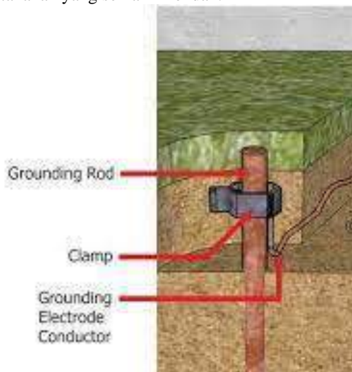
Gambar 2.5 Batang pentanahan disertakan aksesorisnya.
