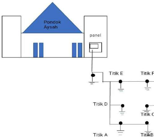
Gambar 4.4. Rancangan perbaikan penanaman grounding
