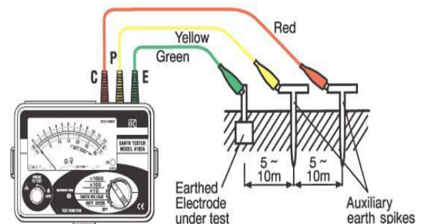
Gambar 2.8 Pengukuran metode 3 kutub
