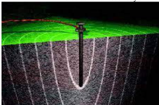
Gambar 2.6 Batang pentanahan dan lingkaran pengaruhnya.
