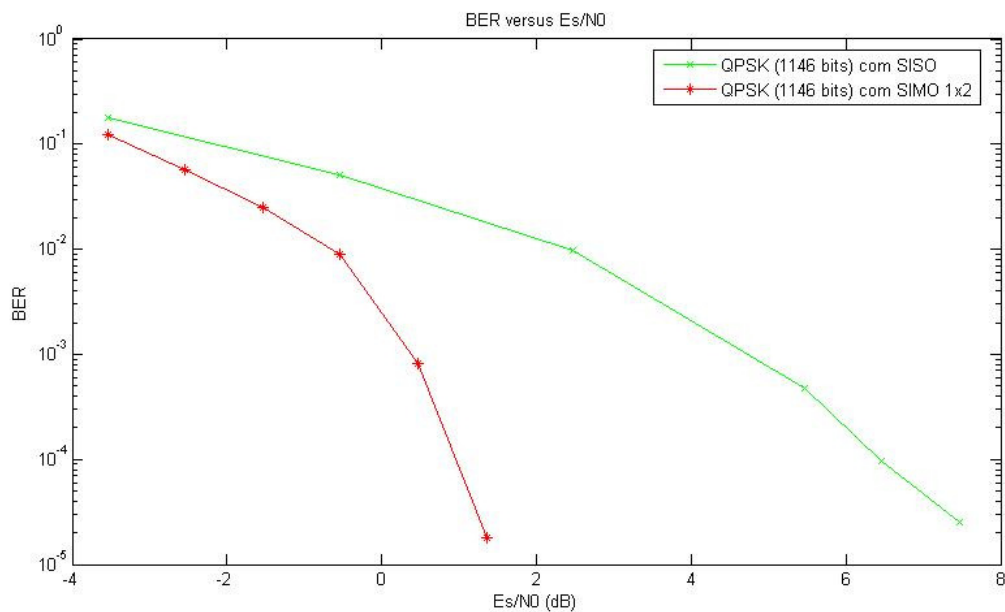
Figura A.2 - Modulação QPSK (1146 bits): com SISO versus com SIMO 1x2
