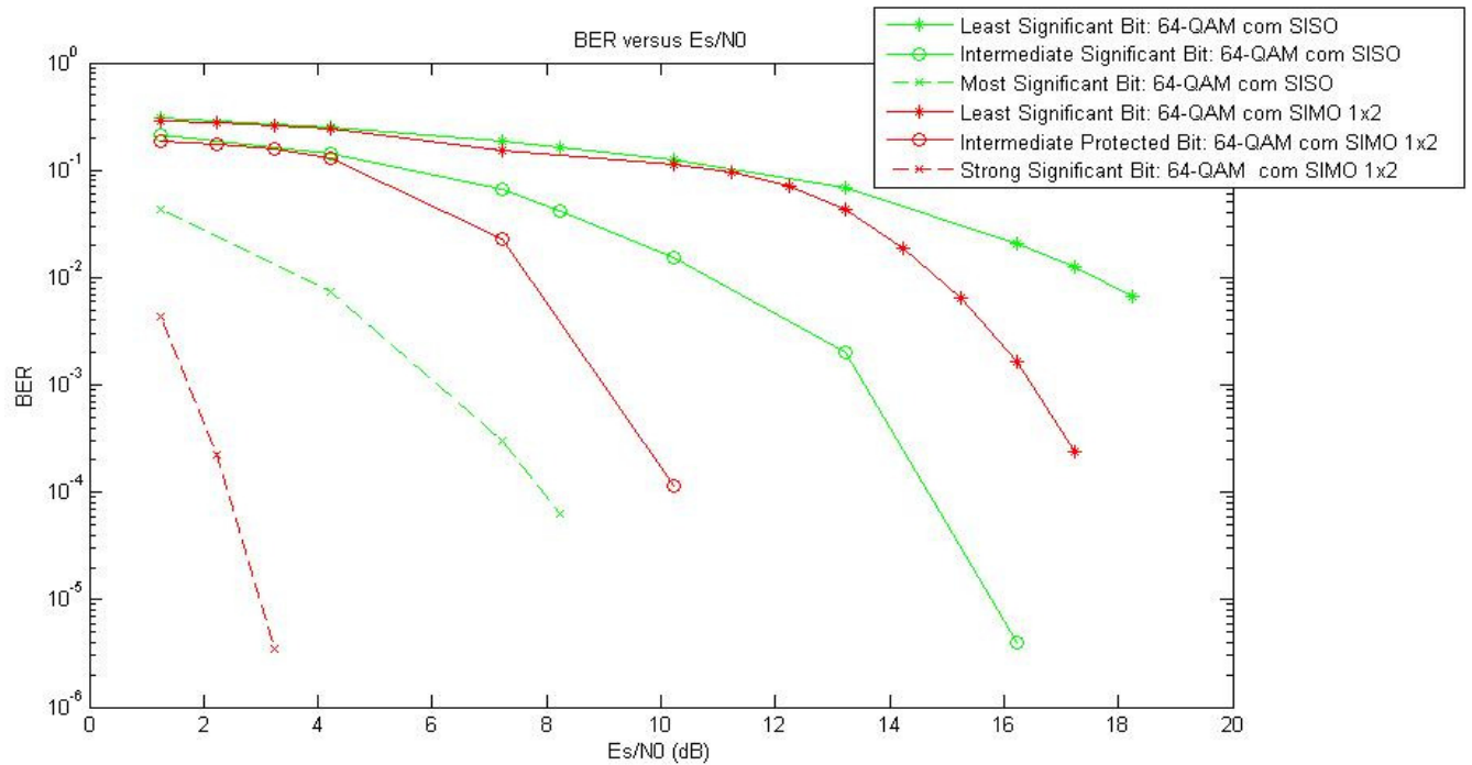
Figura A.10 - Modulação 64-QAM (1146 bits): SISO versus SIMO 1x2
