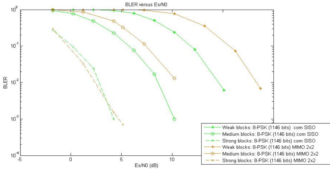
Figura 4.15 - Modulação 8-PSK (1146 bits): SISO versus MIMO 2x2
