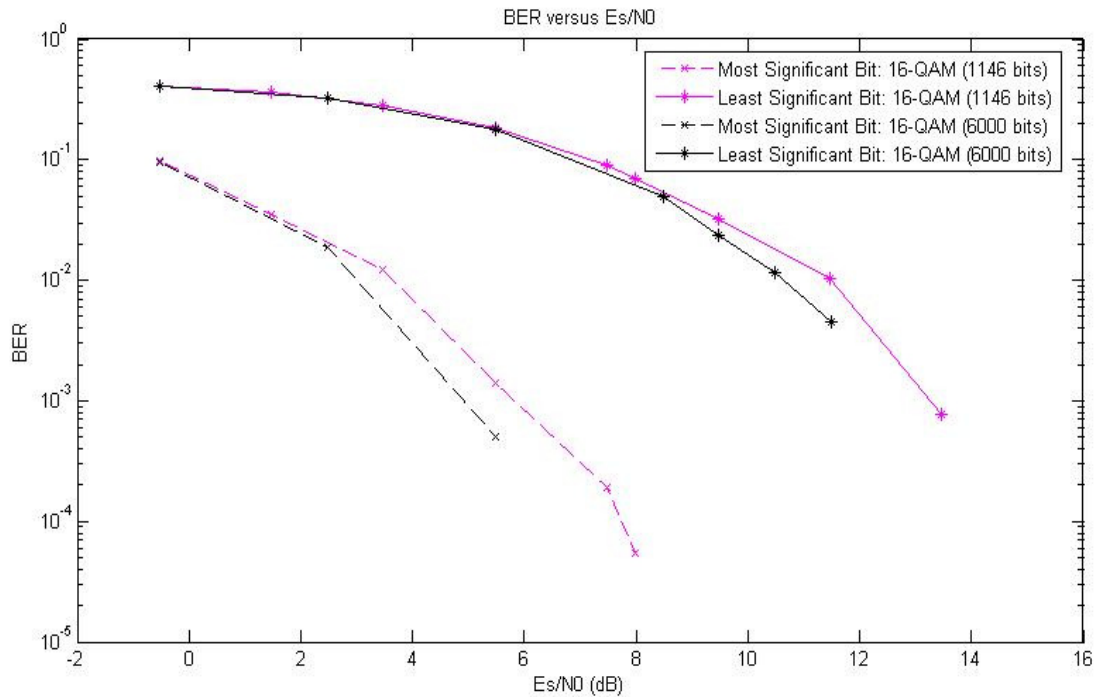
Figura A.5 - Modulação 16-QAM: 1146 bits versus 6000 bits
