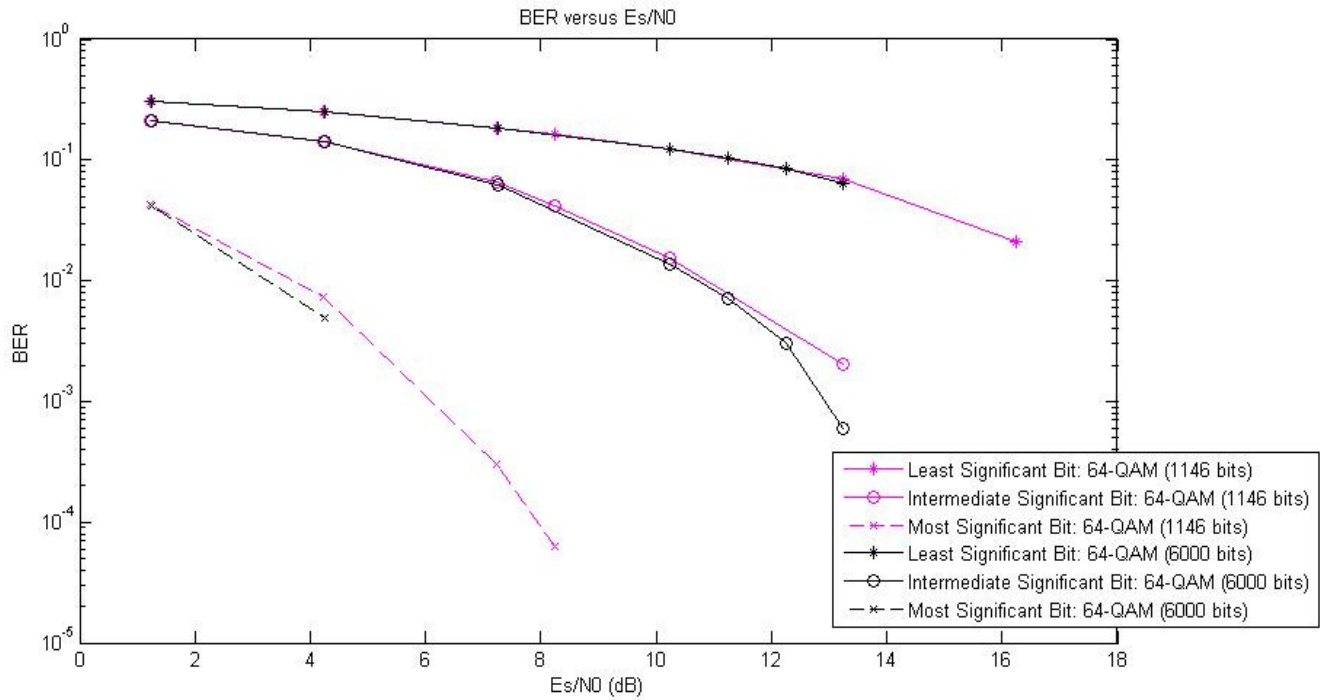
Figura A.9 - Modulação 64-QAM: 1146 bits versus 6000 bits
