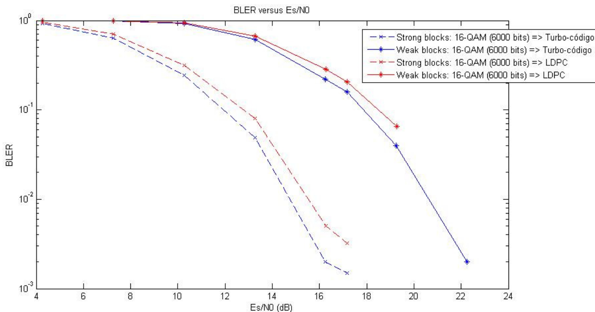
Figura 4.8 - Modulação 16-QAM (6000 bits): turbo-códigos versus LDPC (taxa de código: 2/3)
