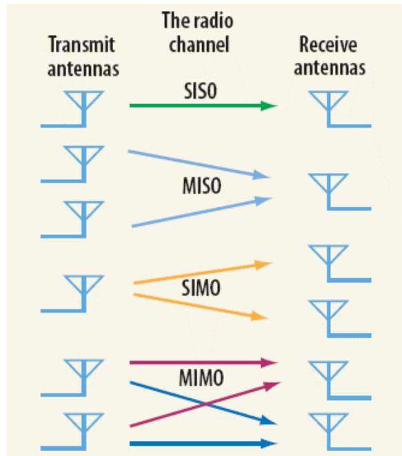
Figura 2.10 - Esquemas SISO, MISO, SIMO e MIMO
