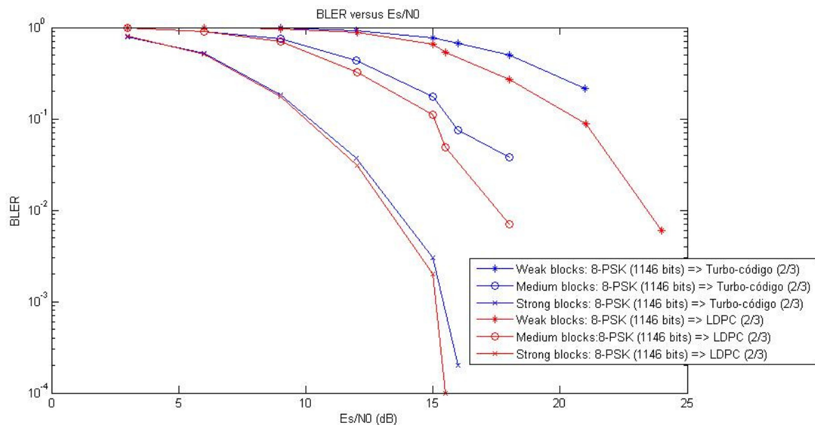
Figura 4.16 - Modulação 8-PSK (1146 bits): turbo-códigos versus LDPC (taxa de código: 2/3)
