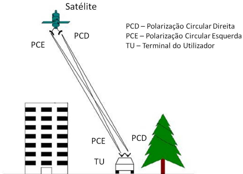
Figura 2.11 - Cenário de Diversidade de Polarização Dupla
