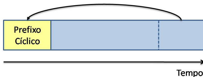
Figura 2.6 - Prefixo Cíclico
