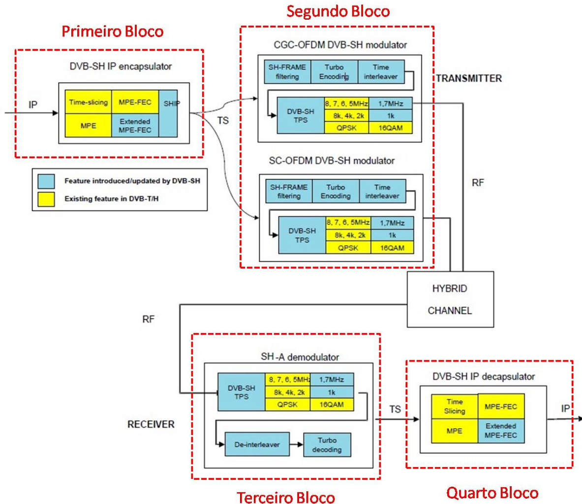
Figura 2.2 - Arquitectura do sistema SH-A
