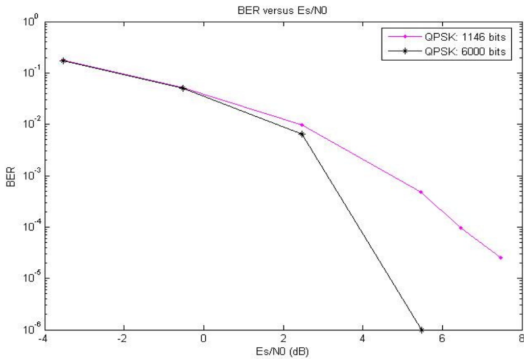
Figura A.1 - Modulação QPSK: 1146 bits versus 6000 bits
