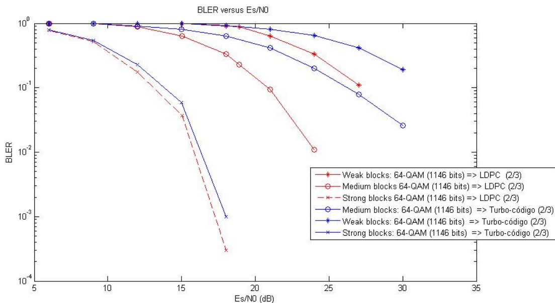
Figura 4.12 - Modulação 64-QAM (1146 bits): turbo-códigos versus LDPC (taxa de código: 2/3)
