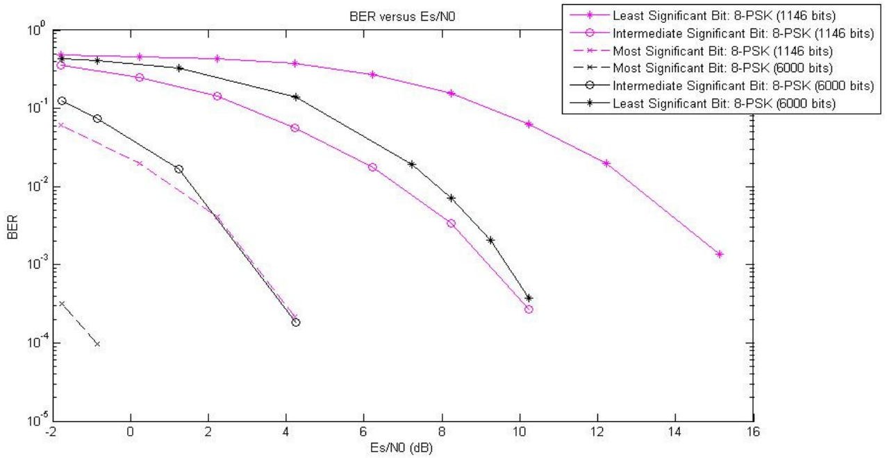
Figura A.13 - Modulação 8-PSK: 1146 bits versus 6000 bits
