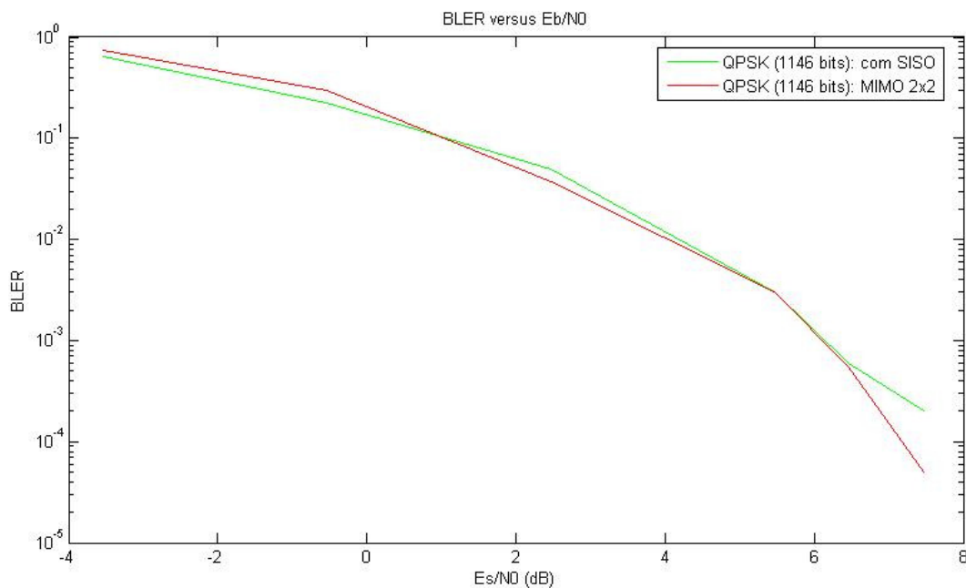
Figura 4.3 - Modulação QPSK (1146 bits): SISO versus MIMO 2x2
