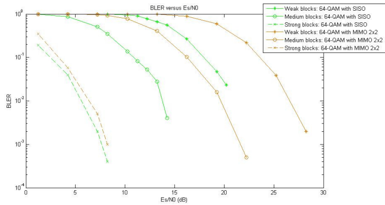
Figure 8 - 64-QAM: SISO versus 2x2 MIMO
