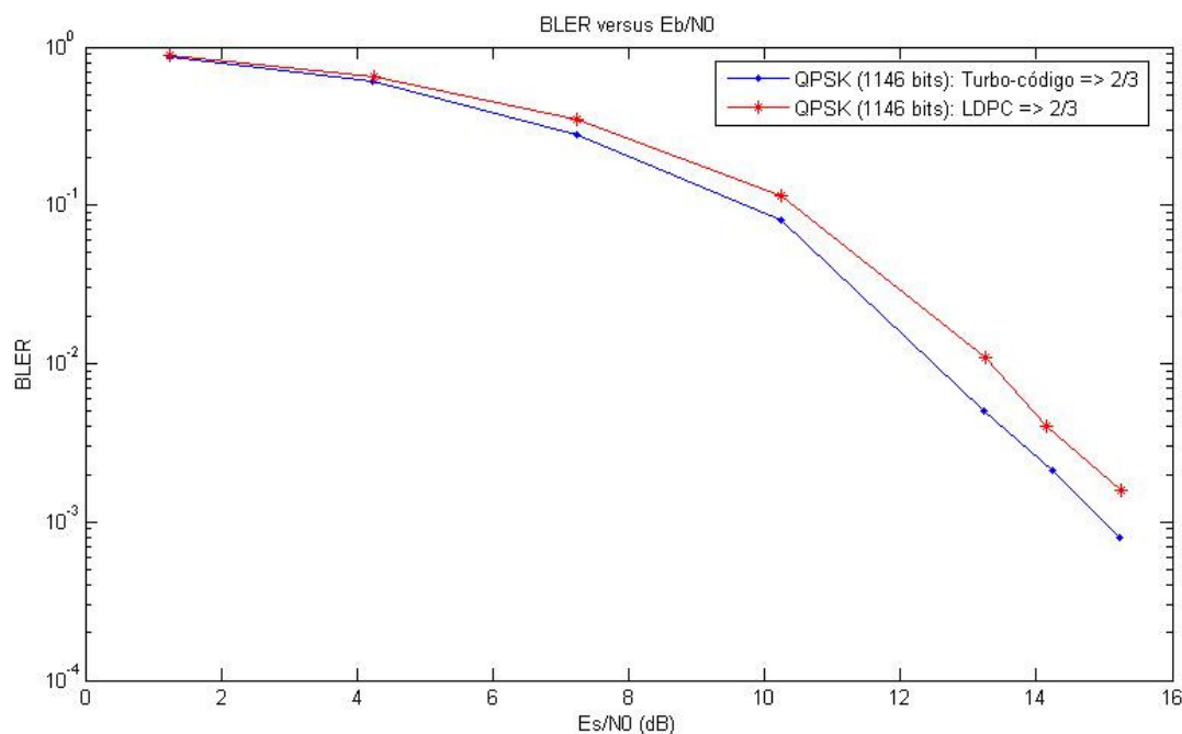
Figura 4.4 - Modulação QPSK (1146 bits): turbo-códigos versus LDPC (taxa de código: 2/3)
