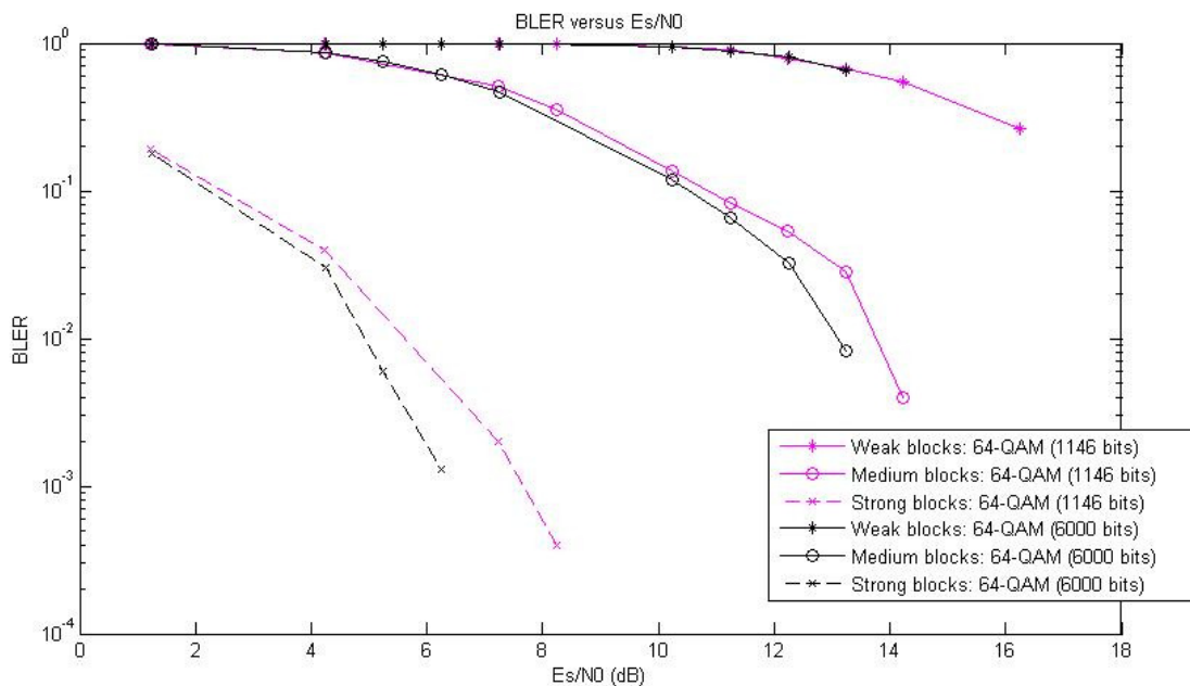
Figura 4.9 - Modulação 64-QAM: blocos de 1146 bits versus blocos de 6000 bits
