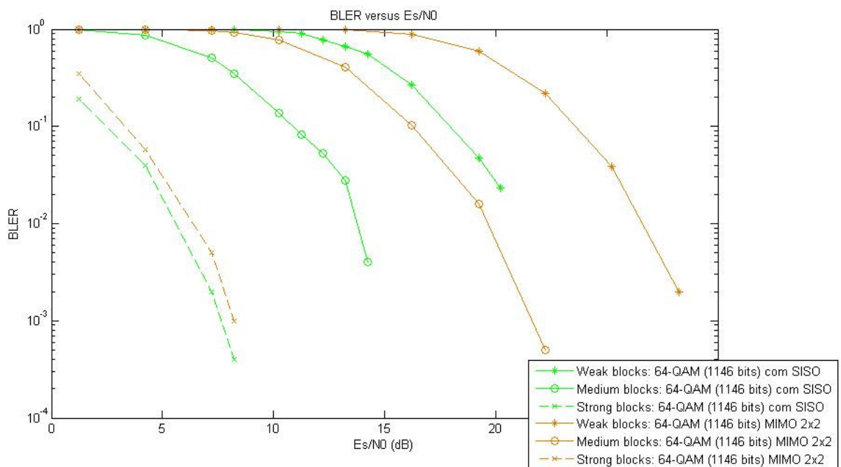
Figura 4.11 - Modulação 64-QAM (1146 bits): SISO versus MIMO 2x2
