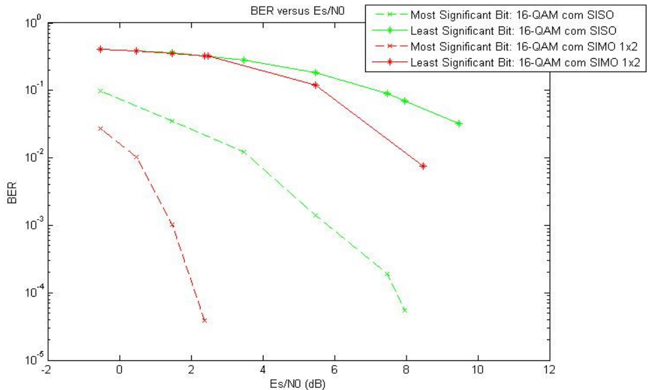
Figura A.6 - Modulação 16-QAM (1146 bits): SISO versus SIMO 1x2
