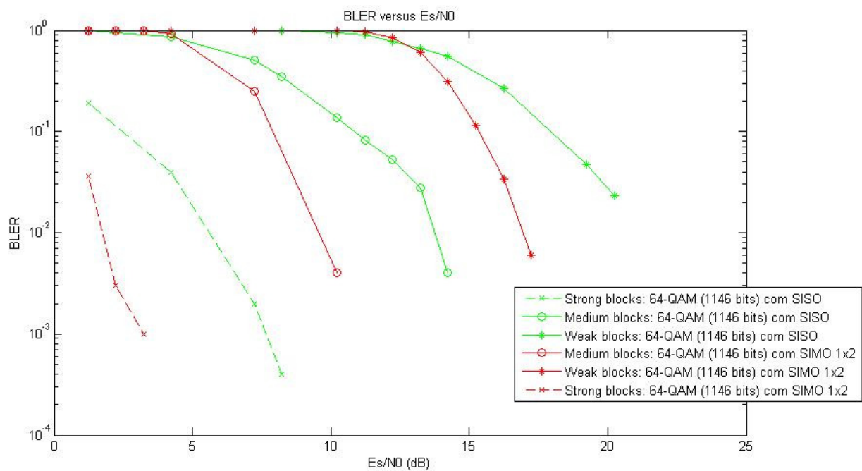
Figura 4.10 - Modulação 64-QAM (1146 bits): SISO versus SIMO 1x2
