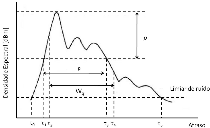
Figura 2.16 - Exemplo de Power Delay Profile [39]
