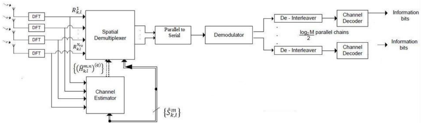
Figura 3.12- Esquema do Receptor
