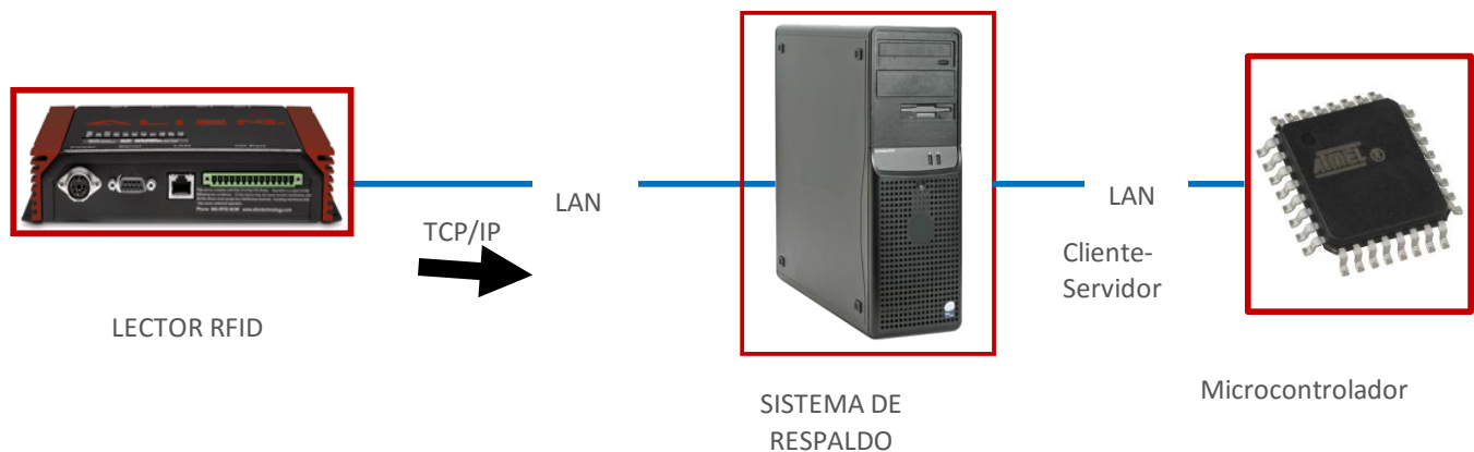
Figura 3. Diagrama de bloques de los protocolos de comunicación.
