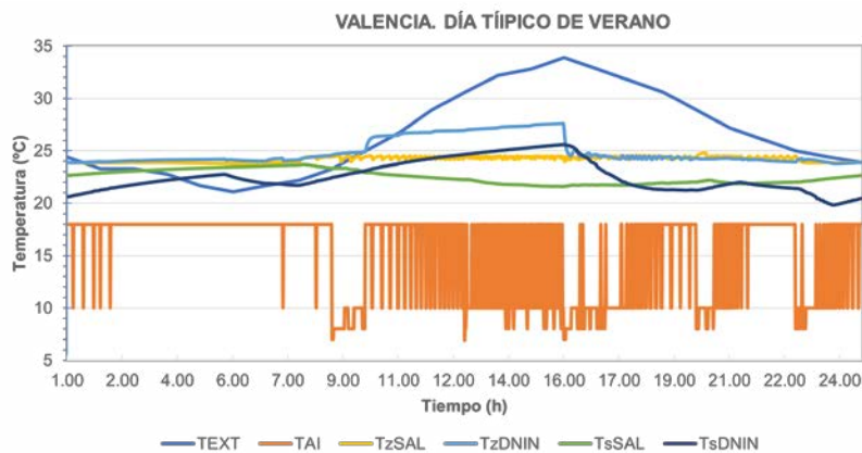
Figura 4. Funcionamiento del sistema para un día de verano en Valencia.
