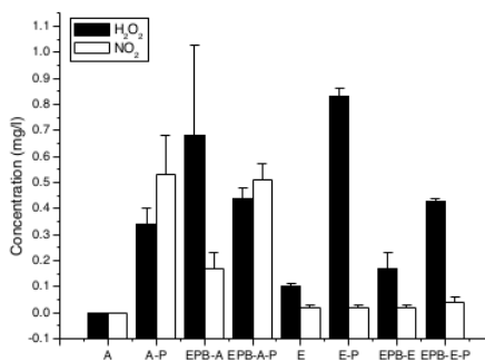
Gambar 6. Konsentrasi H 2 O 2 and NO 2 pada air murni (A), plasma jet dengan air murni (A-P), Ekstrak ethanol sirih dalam air murni (EPB-A), ethanol (E), ekstrak ethanol daun sirih dilarutkan dalam ethanol (EPB-E) dan plasma jet dengan EPB-E (EPB-E-P) (Rahayu et al., 2019). [18].
