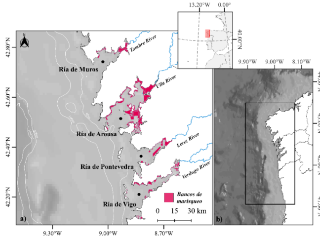
Fig. 1: a) Localización de la zona de estudio. Zonas de marisqueo de R. decussatus , R. philippinarum , V. corrugata y C. edule representadas en color púrpura. b) El rectángulo indica el área modelada.
