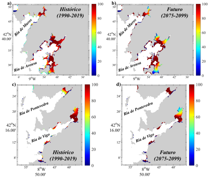
Fig. 3: Índice de confort térmico (TCI, %) para R. philippinarum durante julio-agosto para las rías en el periodo histórico (1990-2019) (a y c) y el periodo futuro (2075-2099) (b y d).
