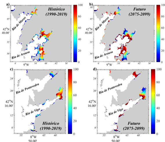
Fig. 5: Índice de confort térmico (TCI, %) para C. edule durante julio-agosto para las rías en el periodo histórico (1990-2019) (a y c) y el periodo futuro (2075-2099) (b y d).
