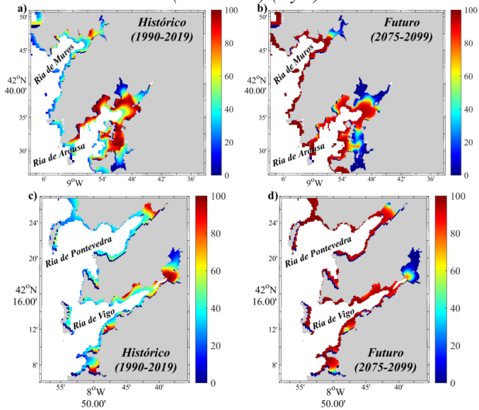
Fig. 4: Índice de confort térmico (TCI, %) para V. corrugata durante julio-agosto para las rías en el periodo histórico (1990-2019) (a y c) y el periodo futuro (2075-2099) (b y d).
