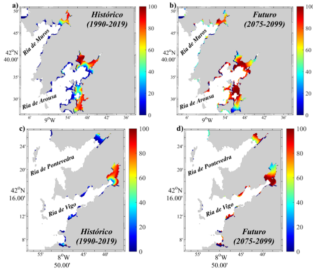
Fig. 2: Índice de confort térmico (TCI, %) para R. decussatus durante julio-agosto para las rías en el periodo histórico (1990-2019) (a y c) y el periodo futuro (2075-2099) (b y d).
