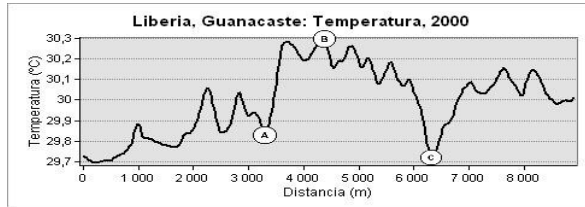
Figura 2. Gráfico de tendencia de temperatura superficial, 2000. Fuente: elaboración propia con datos de imagen landsat
