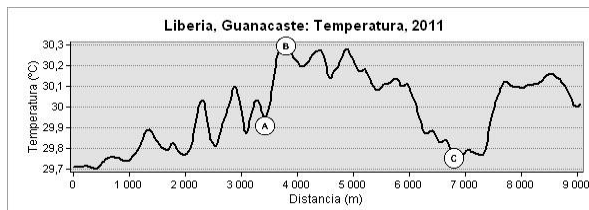
Figura 4. Gráfico de tendencia de temperatura superficial, 2011. Fuente: elaboración propia con datos de imagen landsat
