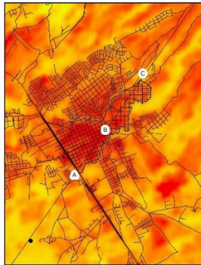
Figura 5. Temperatura superficial, 2019. Fuente: elaboración propia con datos de imagen landsat
