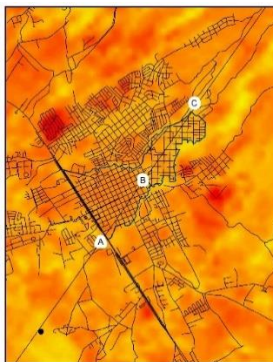
Figura 1. Temperatura superficial, 2000. Fuente: elaboración propia con datos de imagen landsat
