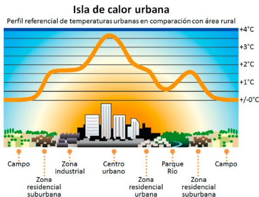
Figura 7. Perfil referencial de temperaturas urbanas en comparación con áreas rurales por la isla de calor. Fuente: Periódico Arquitectura y Energía. (2015).
