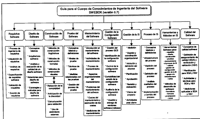
Figura 1. Descomposición temática de SWEBOK (versión Stoneman)
