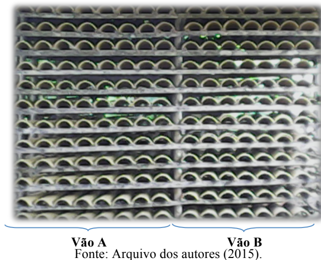
Figura 3 - Vãos construídos pelos oleiros com as telhas para secagem
