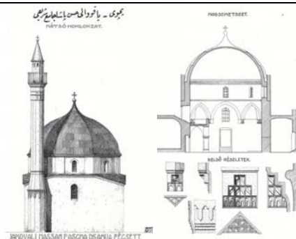
1. ábra. A dzsámi homlokzata és metszete Faerk Ernő felmérésén, 1917. [7]
