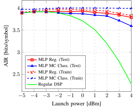
(d) TWC link - MLP Equalizer - AIR Metric
