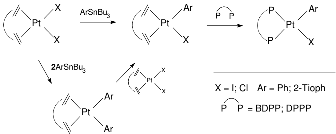
3. ábra: Pt(PP)(X)(alkil/aryl) típusú komplexek előállítása
