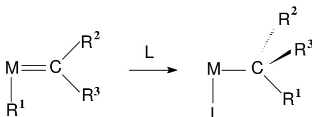
1. ábra: Aszimmetriacentrum kialakulása karbén-beékelődés során.
