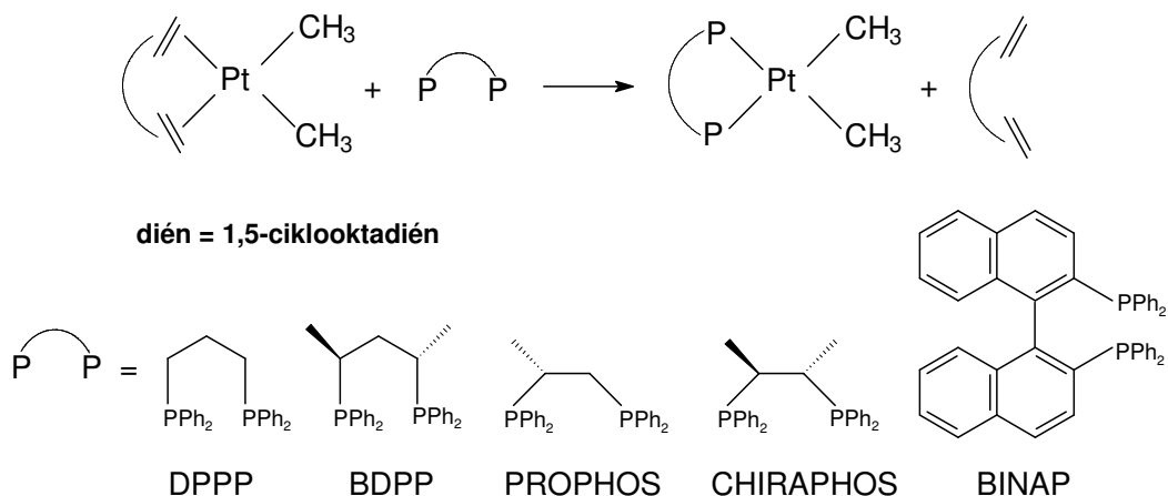
2. ábra: Platina-dimetil-COD-komplex ligandumcserés reakciója, valamint a felhasznált difoszfín ligandumok
