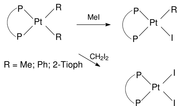
4. ábra: Pt{(S,S)-BDPP}(I)(R) (R = Me, Ph, 2-Tioph) típusú komplexek előállítása
