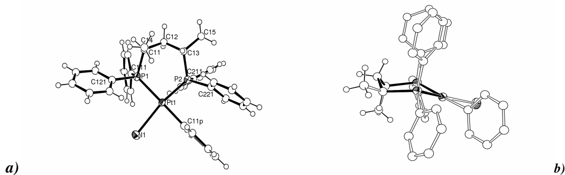
5. ábra: Pt\{(2S,4S)\text{-BDPP}\}(Ph)I komplex ORTEP diagrammja: (a) felülnézeti képen a ligandumok síknégyzetes elhelyezkedését láthatjuk a központi platina fém körül., (b) odalnézet a kelát gyűrű szék konformációját mutatja
