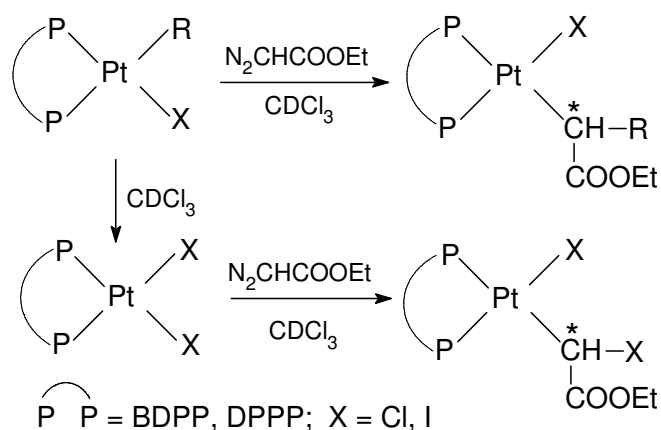
6. ábra: Etil-diazoacetátból képződő karbén inzerciója platina-aril, valamint platina-halogén kötésbe, a Pt(P-P)(X)(R) típusú komplexek esetében ( R = Ph, 2\text{-Tioph} ).
