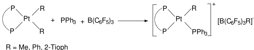
7. ábra: [\text{Pt}(\text{BDPP})(\text{alkil/aril})(\text{PPh}_3)]^+ komplexek képződése
