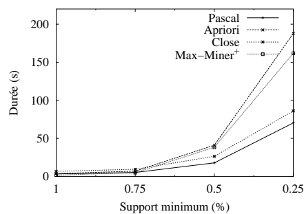
Figure 8. Résultats expérimentaux pour T25I10D10K
