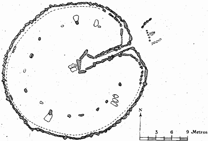
Fig. 13 — Sepulcro de corredor de Bryn Celli Ddu (Grupo de Anglesey)
