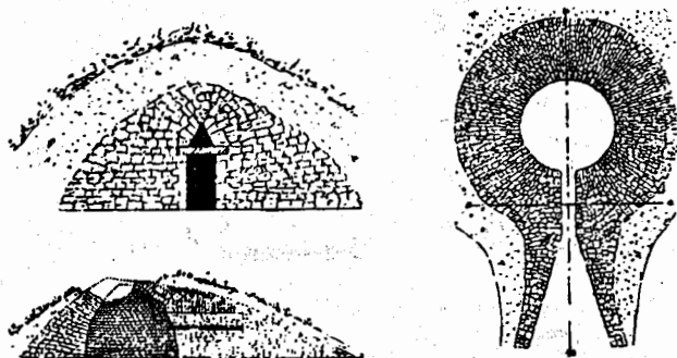
Fig. 3 — Tholos sepulcral micênico, da Ilha de Eubea (Grécia)
