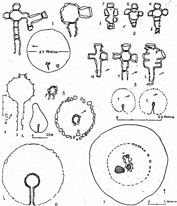
Fig. 12— Sepulcros de corredor irlandeses
