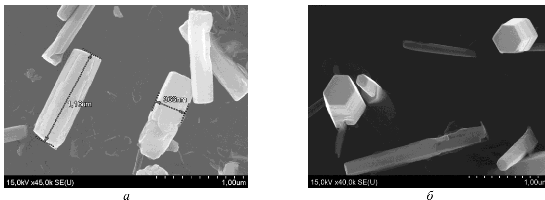
Рис. 2. Электронные фотографии легированных нанокристаллов оксида цинка, сформированных гидротермальным методом на подложках монокристаллического кремния электронного типа проводимости в растворе, содержащем 0,1 М Zn(NO_3)_2 , 0,1 М C_6H_{12}N_4 и 0,001 М Al(NO_3)_3 при температуре 85°С (а) и 95°С (б); время осаждения для всех образцов 120 мин
