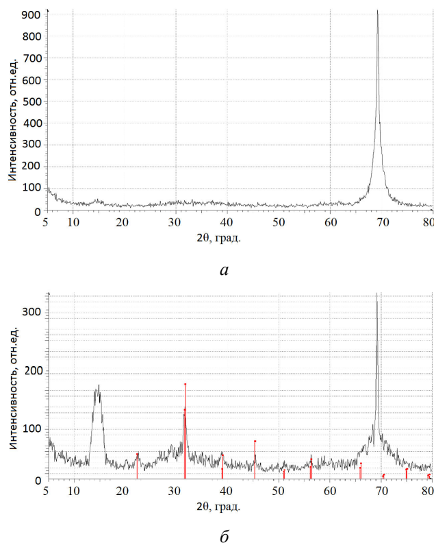
Рис. 2. Дифрактограмма пленок ВаТiО 3 на кремнии после термообработки при температуре 850 °С: а – однослойная пленка; б – пятислойная пленка
