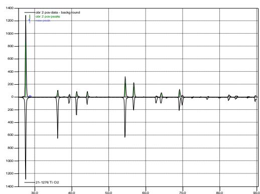
Рис. 3. Сравнение рентнограмм поверхности исследуемого образца и эталонных карточек: a – рентнограмма образца; б – эталонные карточки \text{TiO}_2 , \text{Ti}_2\text{N}
