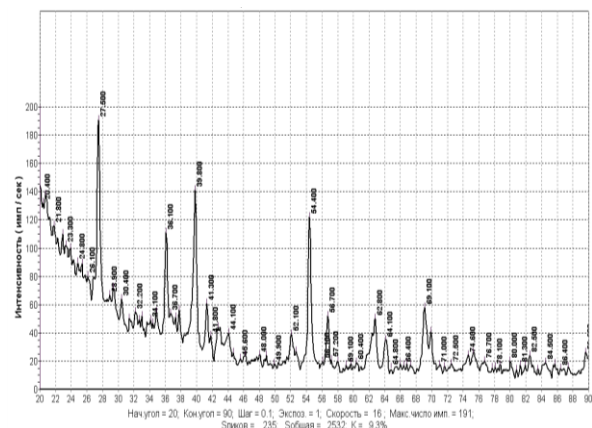
Рис. 4. Рентнограмма в глубине образца
