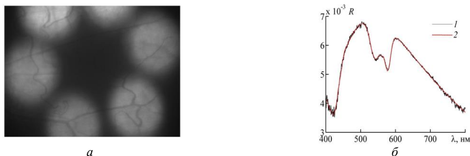
Рис. 1. Результаты измерения спектра обратного рассеяния света конъюнктивой добровольца: a – изображение светящегося торца волоконно-оптического датчика в плоскости конъюнктивы, б – измеренный спектр (1) и результат его подбора в рамках разработанной модели (2)
