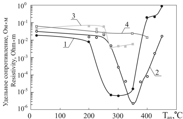
Рис. 4. Зависимость удельного сопротивления от температуры отжига пленок оксида ванадия, нанесенных при различной концентрации кислорода в Ar/O 2 смеси газов:
