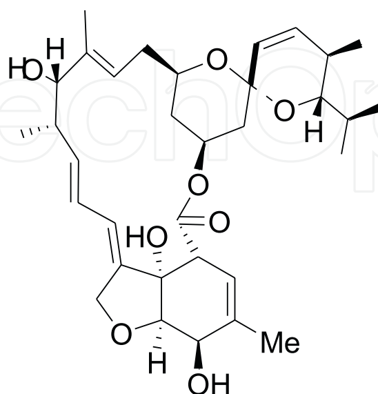
Emamectin Scaflod
