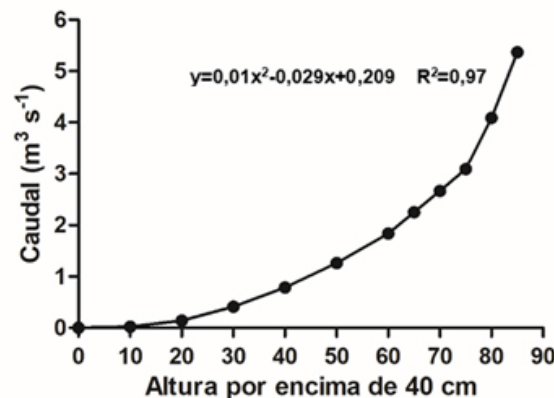
Figura 2. Curva de caudal (q) vs altura de agua registrada por encima del sensor del limnógrafo (h=40 cm).
