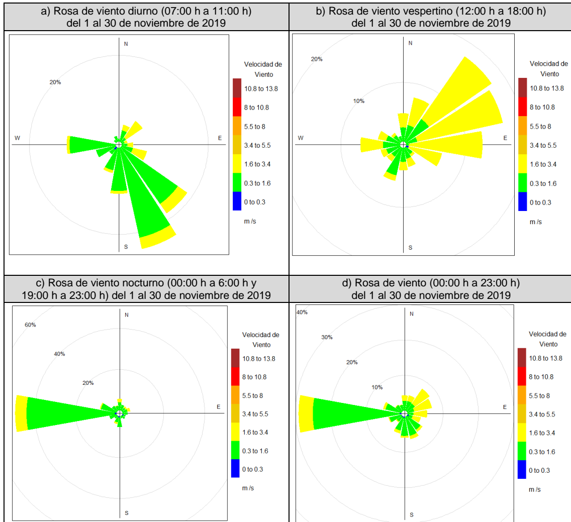
Figura 5.1. Representación gráfica de las rosas de vientos en la estación de vigilancia ambiental CA-CC-01, en noviembre de 2019 a) en horario diurno, b) en horario vespertino, c) en horario nocturno, d) en todas las horas del mes.
