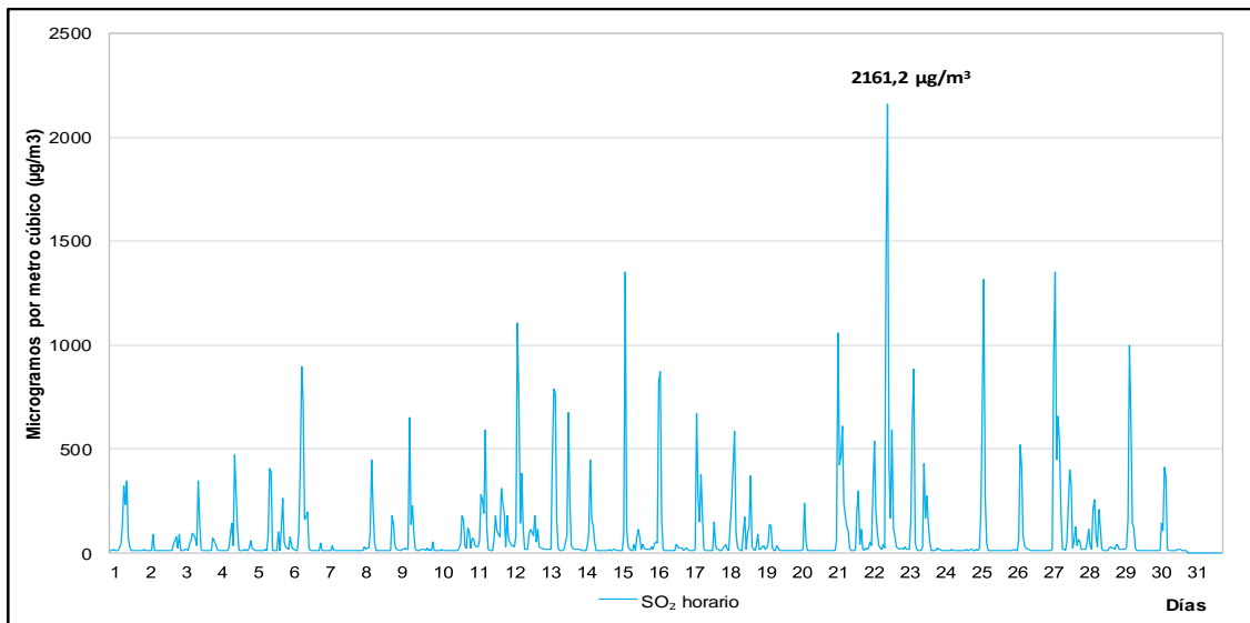
Figura 5.4. Concentraciones horarias de SO 2 en la estación de vigilancia ambiental CA-CC-01 en noviembre de 2019.
