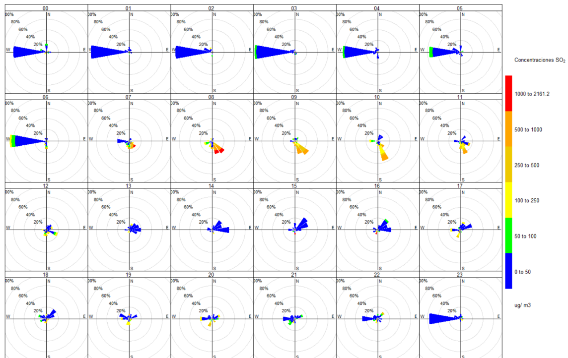
Figura 5.5. Rosas de concentración por horas para el SO 2 en la estación de vigilancia CA-CC-01, desde las 00:00 horas hasta las 23:00 horas en noviembre de 2019 Nota: Las paletas indican la dirección de donde provienen las concentraciones de SO 2 .
