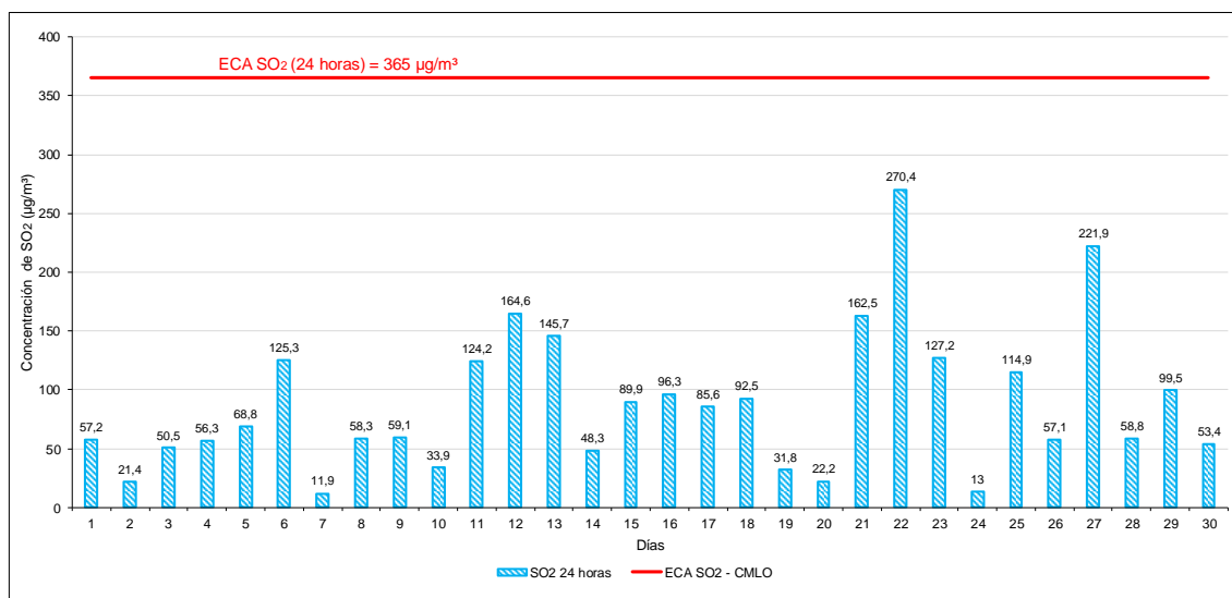
Figura 5.3. Concentraciones de 24 horas de SO 2 en la estación de vigilancia ambiental CA-CC-01, en noviembre de 2019
