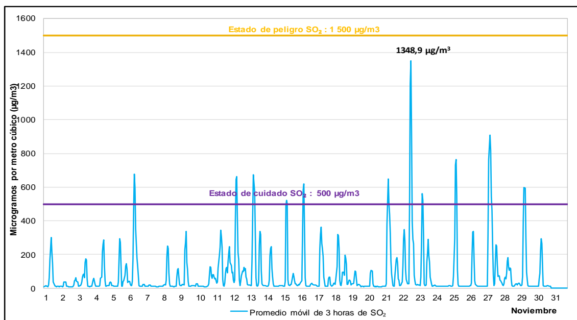
Figura 5.6. Promedio móvil de 3 horas de la concentración de SO 2 comparados con los niveles de estado de alerta establecidos en D.S. N.º 009-2003-SA y modificatoria D.S. N.º 012-2005-SA, en la estación de vigilancia ambiental CA-CC-01 correspondiente a noviembre de 2019
