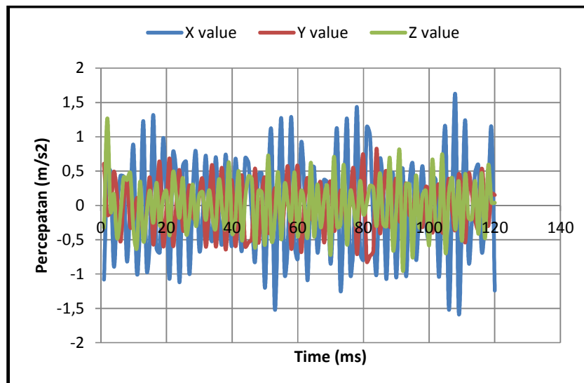
Gambar 4. 2 Grafik Pengujian Parameter Getaran pada Footrest Sepeda Motor Matic (Beat)
