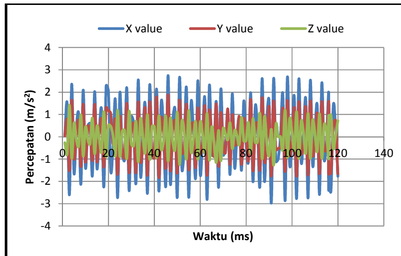
Gambar 4. 1 Grafik Pengujian Parameter Getaran pada Footrest Sepeda Motor Non-Matic (Vega Zr)
