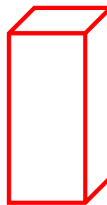
Gambar 13. Balok
