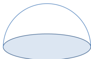
Gambar 3. Setengah Bola
