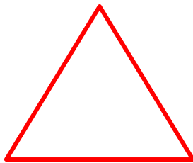
Gambar 11. Segitiga
