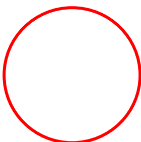
Gambar 7. Lingkaran
