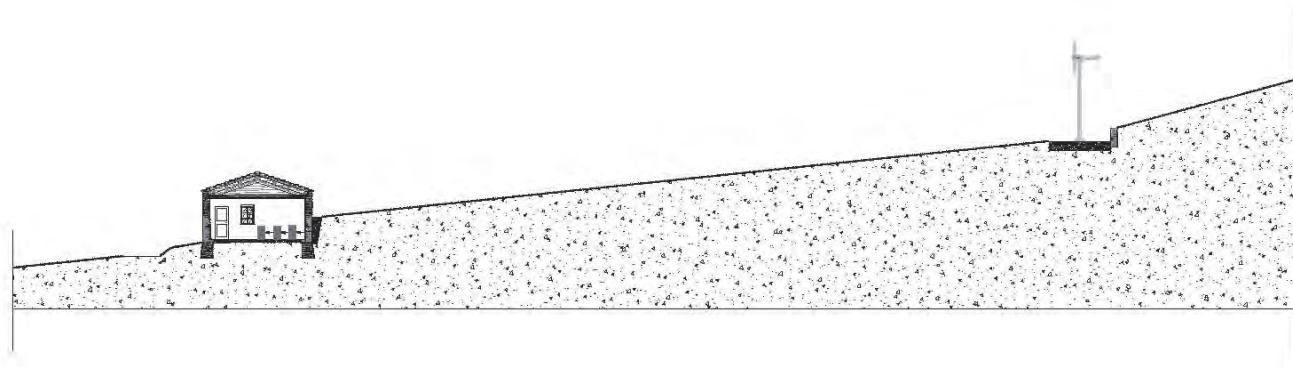
Schema di impianto micro-eolico
