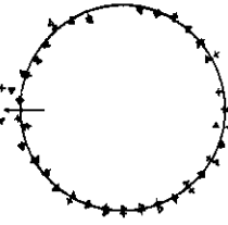
図 19 「曲げばね」実験 P3-4.5-80 の各加振振動数 (30 Hz から 21 Hz) における円周方向歪の断面分布 Fig. 19 Circumferential Strain Section Distribution of Sinusoidal Excitation (30 Hz-21 Hz) in Test Case P3-K4.5-80
