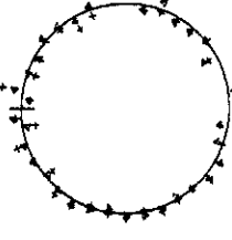
図 19 「曲げばね」実験 P3-4.5-80 の各加振振動数 (30 Hz から 21 Hz) における円周方向歪の断面分布 Fig. 19 Circumferential Strain Section Distribution of Sinusoidal Excitation (30 Hz-21 Hz) in Test Case P3-K4.5-80
